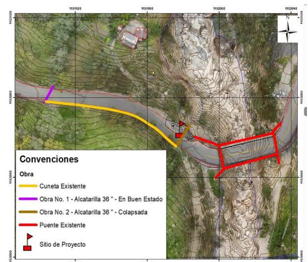
Figura 36. Localización general – Obras de drenaje existentes (Tomado de G&C)
