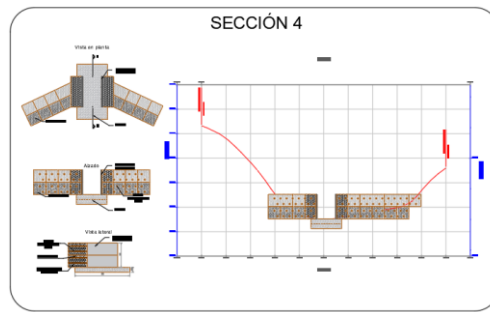
Secciones diques semilleros
