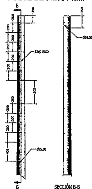
Figura 3. Cima de los postes de 12 m
