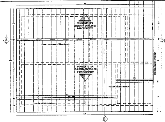
PLANTA ARQUITECTÓNICA CUBIERTA Escala 1:50
