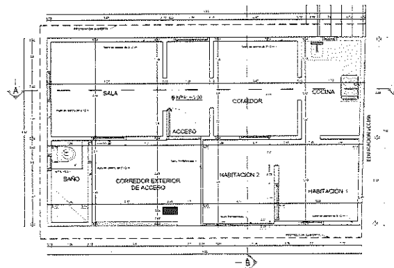
PLANTA ARQUITECTÓNICA PRIMER NIVEL Escala 1:50
