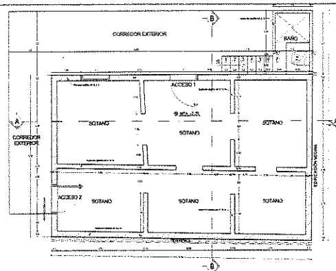
PLANTA ARQUITECTÓNICA SÓTANO Escala 1:50
