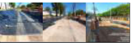
HITO 4 RUTA 7805 PAVIMENTO RÍGIDO COLOCACION DE GEOTEXTIL Y LLENADO CON MATERIAL GRANULAR (AFIRMADO).
