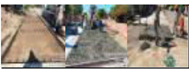
HITO 4 RUTA 7805 PAVIMENTO RÍGIDO FUNDIDA DE LOSAS.
