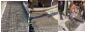
HITO 3 MOMPOIX - GUAMAL RUTA 7804 PAVIMENTO RÍGIDO DE GUAMAL- FIGURACIÓN DE ACERO Y FUNDIDA DE LOSAS EN CONCRETO MR-45.
