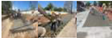
HITO 4 RUTA 7805 PAVIMENTO RÍGIDO FUNDIDA DE LOSAS.
