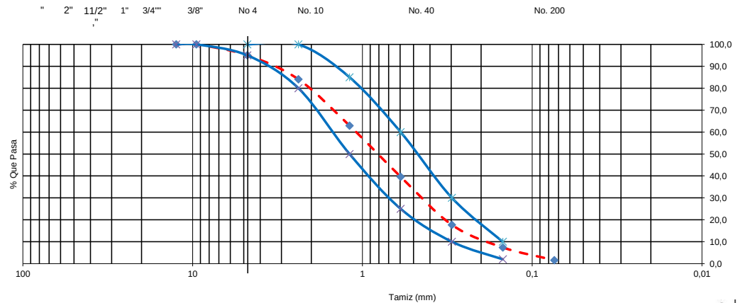
CURVA GRANULOMETRICA
