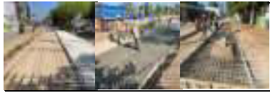
HITO 4 RUTA 4313 PAVIMENTO RÍGIDO - FIGURACIÓN DE ACERO Y FUNDIDA DE LOSAS
