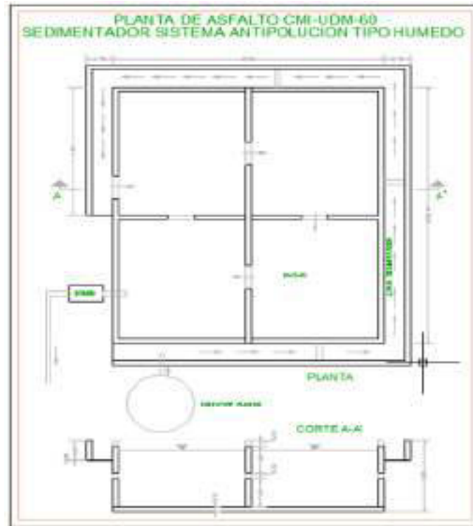
Imagen No. 4: Sistema de antipolución tipo húmedo
