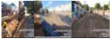
HITO 4 RUTA 7805 PAVIMENTO RÍGIDO EL BANCO - EXCAVACIÓN, RETIRO DE MATERIAL, COLOCACION DE GEOTEXTIL Y POLIETILENO, LLENADO CON MATERIAL GRANULAR (AFIRMADO) Y EXTENDIDO DE SUELOCEMENTO.
