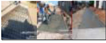
HITO 4 RUTA 7805 PAVIMENTO RÍGIDO - FIGURACIÓN DE ACERO Y FUNDIDA DE LOSAS EN CONCRETO MR-45.
