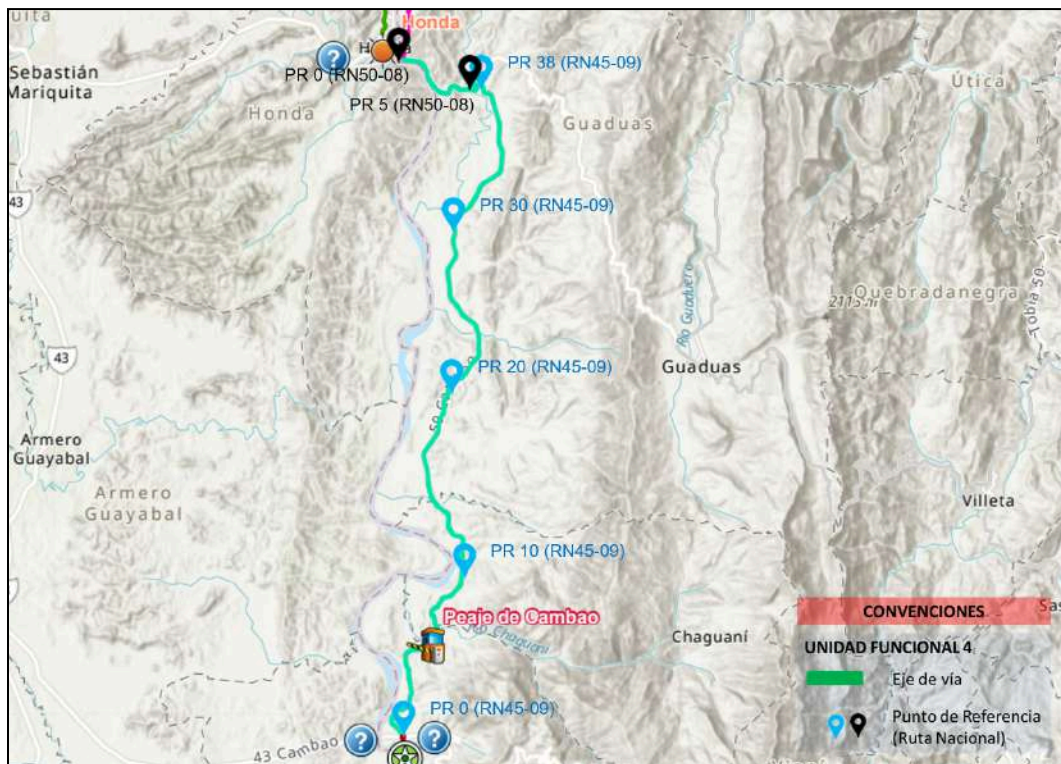
Figura 14. Esquema General Unidad Funcional 5 Fuente: Página Web Concesión Alto Magdalena y Propia
