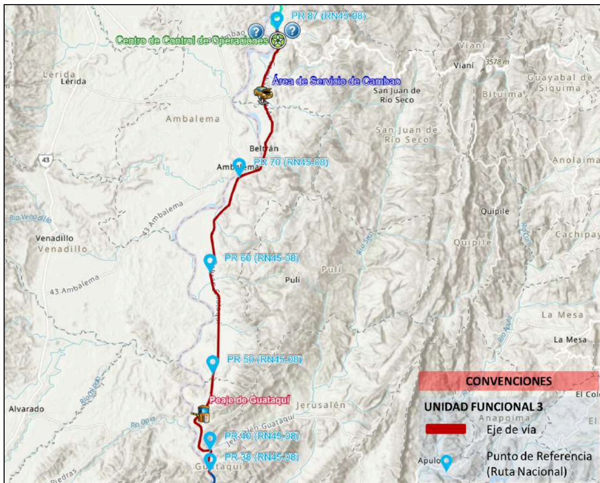
Figura 13. Esquema General Unidad Funcional 3 Fuente: Página Web Concesión Alto Magdalena y Propia
