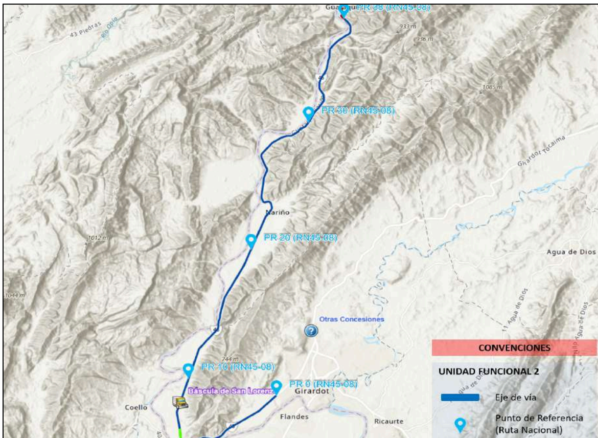
Figura 12. Esquema General Unidad Funcional 2 Fuente: Página Web Concesión Alto Magdalena y Propia
