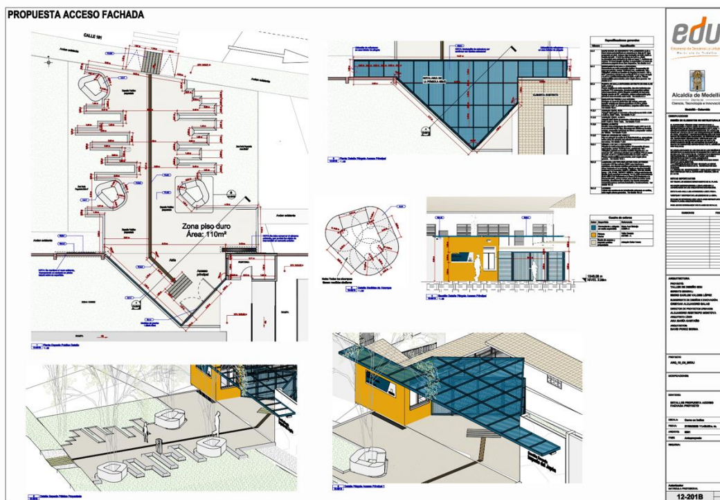
Ilustración 5. Planimetría detalles propuesta de acceso en fachada
