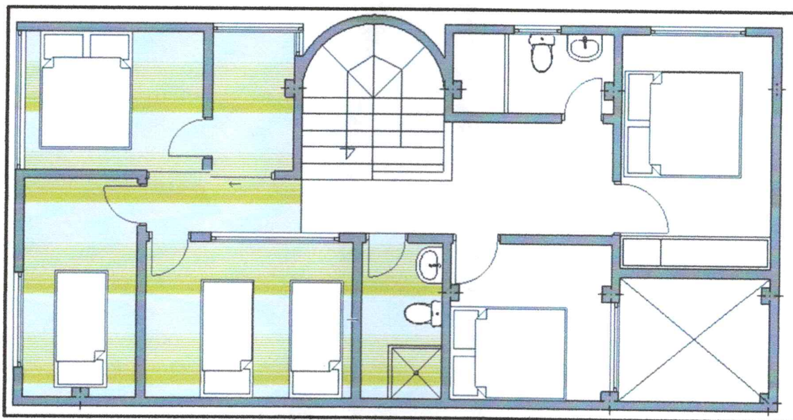
Figura 9. Intervención planta tercer nivel
