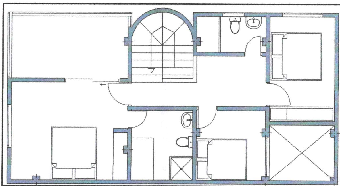
Figura 3. Distribución actual planta tercer nivel
