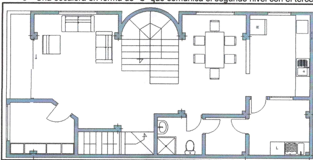
Figura 2. Distribución actual planta segundo nivel
