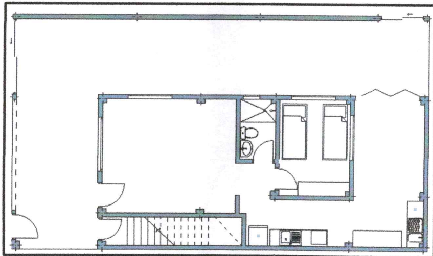
Figura 1. Distribución actual planta primer nivel
