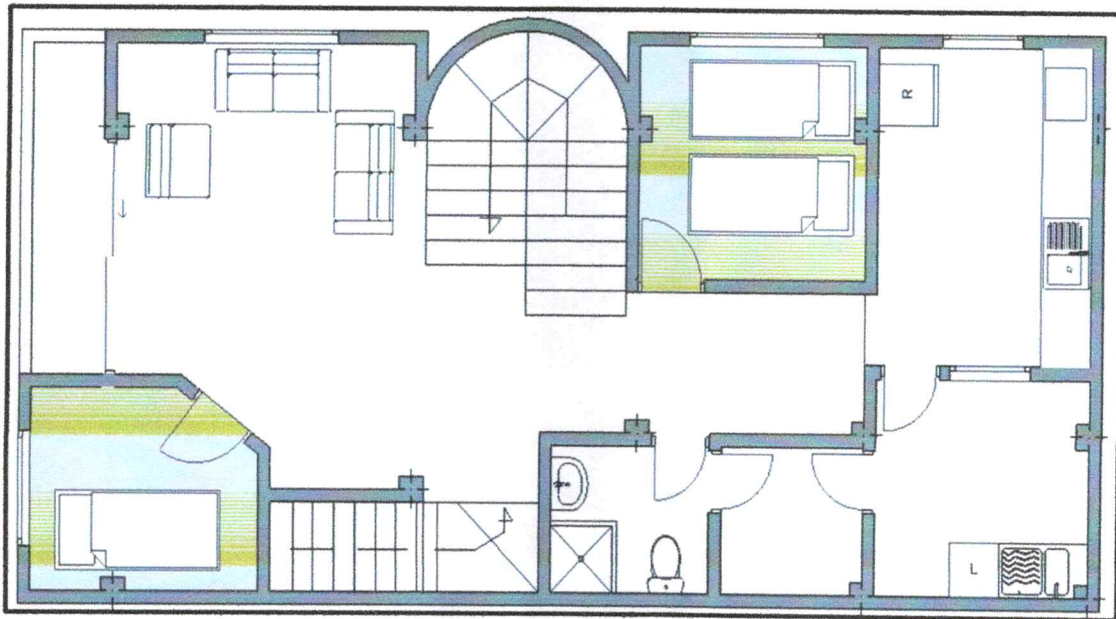
Figura 8. Intervención planta segundo nivel
