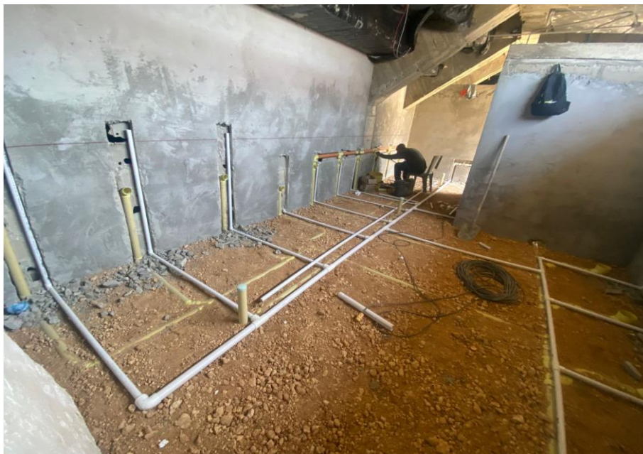
Ilustración 23. Instalaciones hidráulicas baños graderías de futbol
