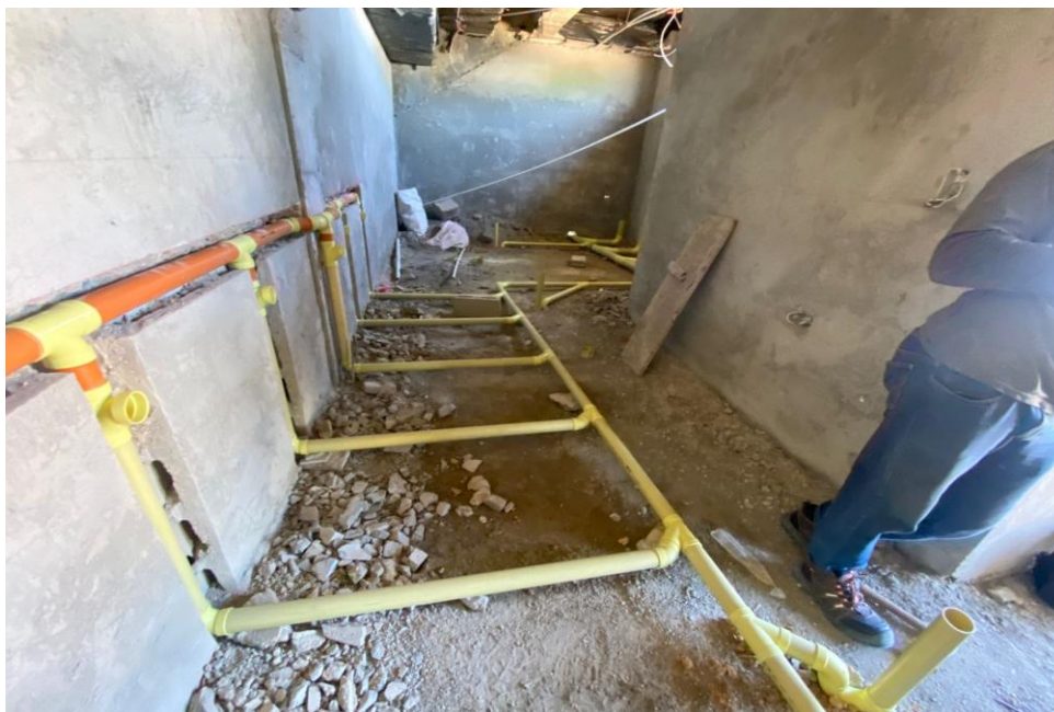
Ilustración 22. Instalaciones sanitarias baños graderías de futbol
