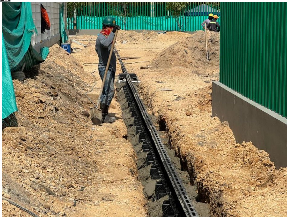
Ilustración 37. Instalación sistema de drenaje aguas lluvias(canaleta)
