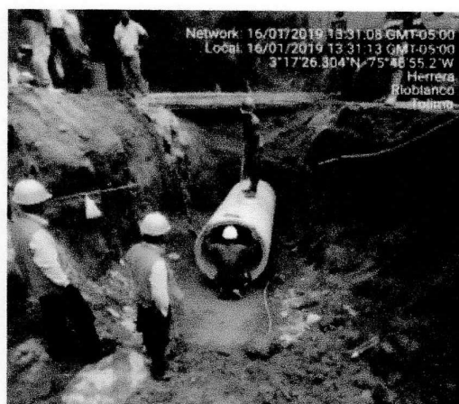
INSTALACION DE TUBERIA PR0+290
