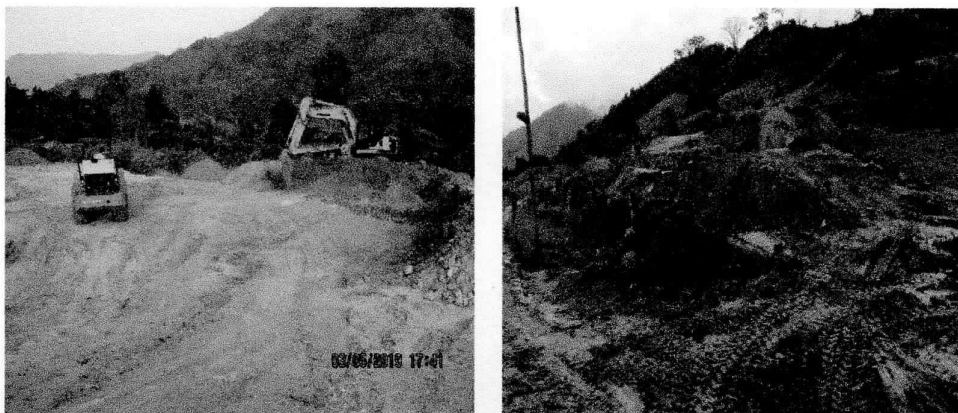
Conformación de talud y terraceo. PR 1 + 500
