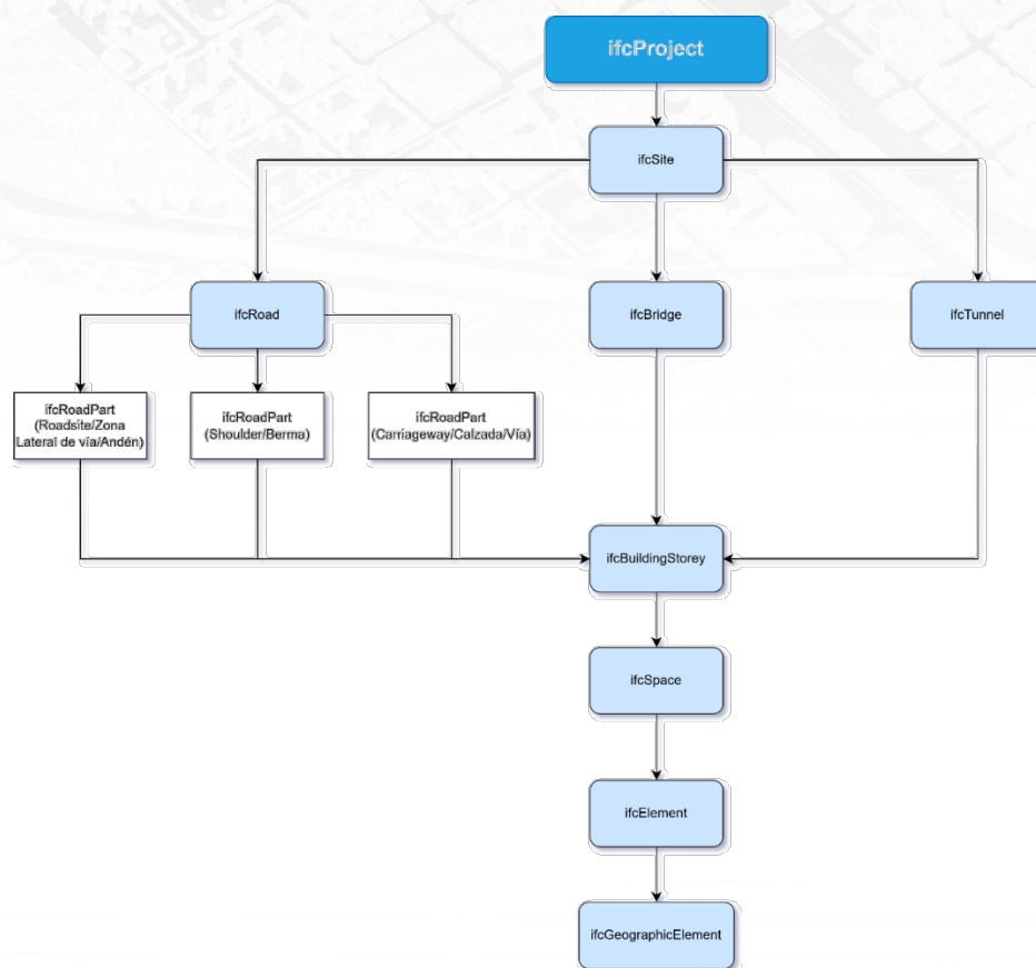
Figura 3. Ejemplo de esquema de estructura de IFC.
