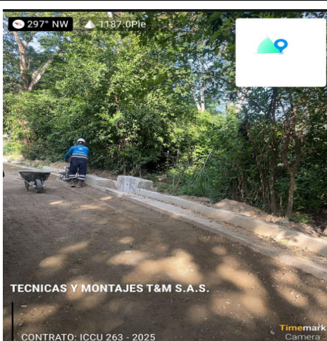
Fotografía 8: Actividades de cunetas
