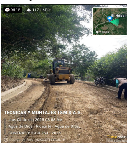
Fotografía 6: Instalación y compactación de Base Granular
