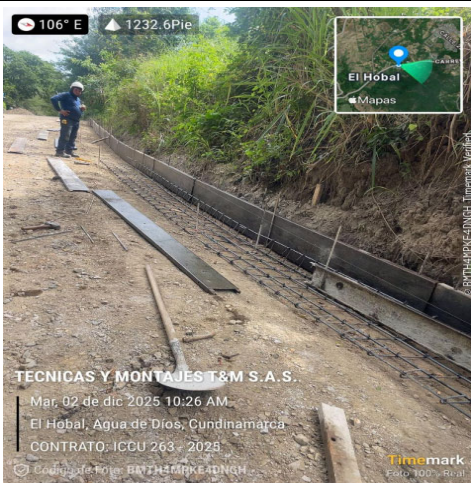
Fotografía 7: Actividades de cunetas
