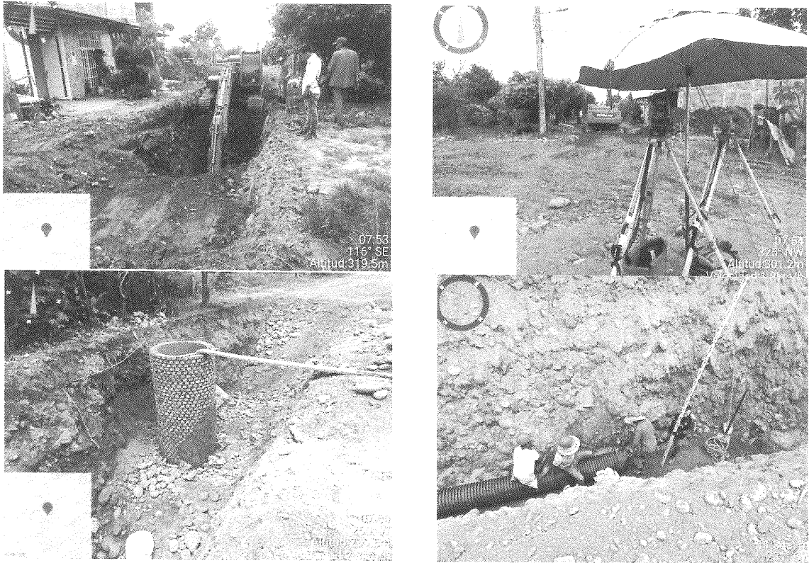
CONSTRUCCIÓN DE COLECTORES Y POZOS DE LA RED DE ALCANTARILLADO SANITARIO
