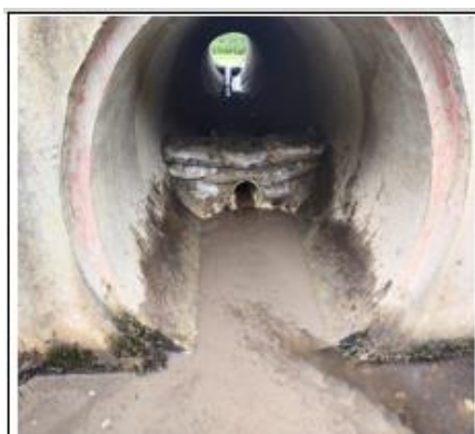
PK 142+470 INSTALACION DE BOLSA CRETO
