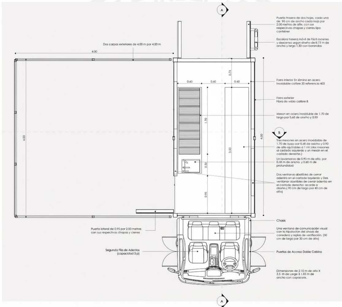
1 Planta de detalle Esc 1 : 25
