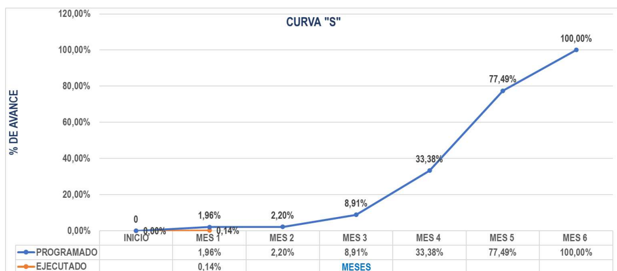
FIGURA 3. Curva "S"
