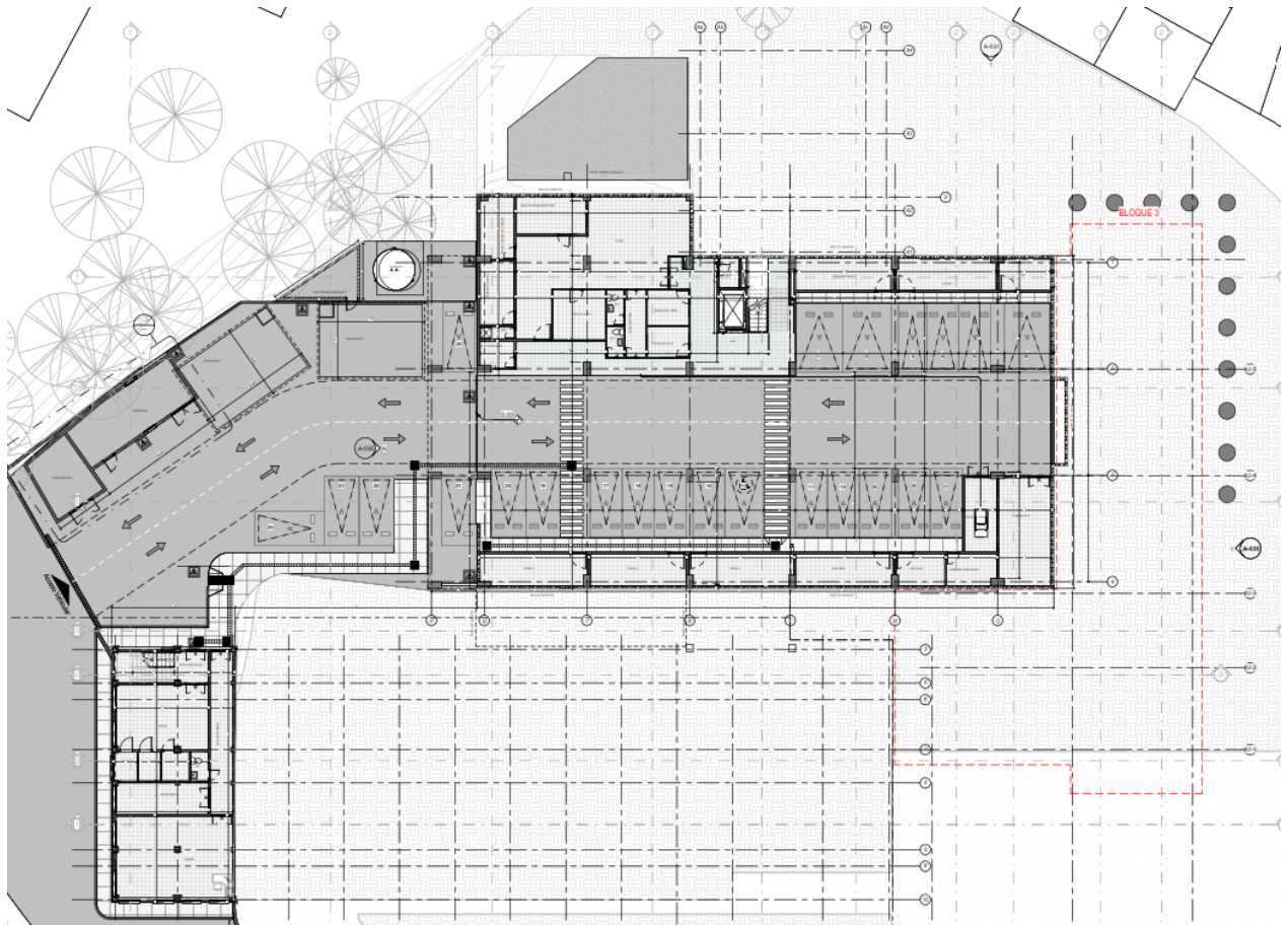
Planta Cubiertas
