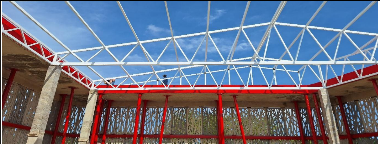
ESTRUCTURA METÁLICA COMPUESTA POR VIGAS EN PERFIL DE ALMA LLENA HEA
