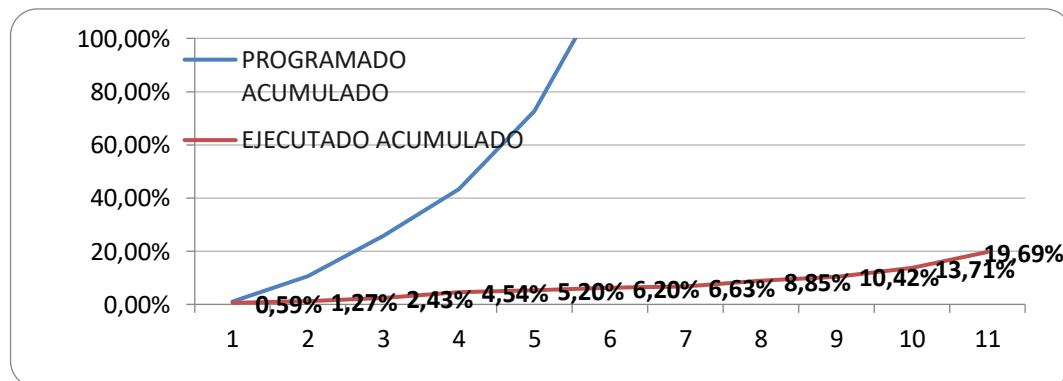
Curva S
