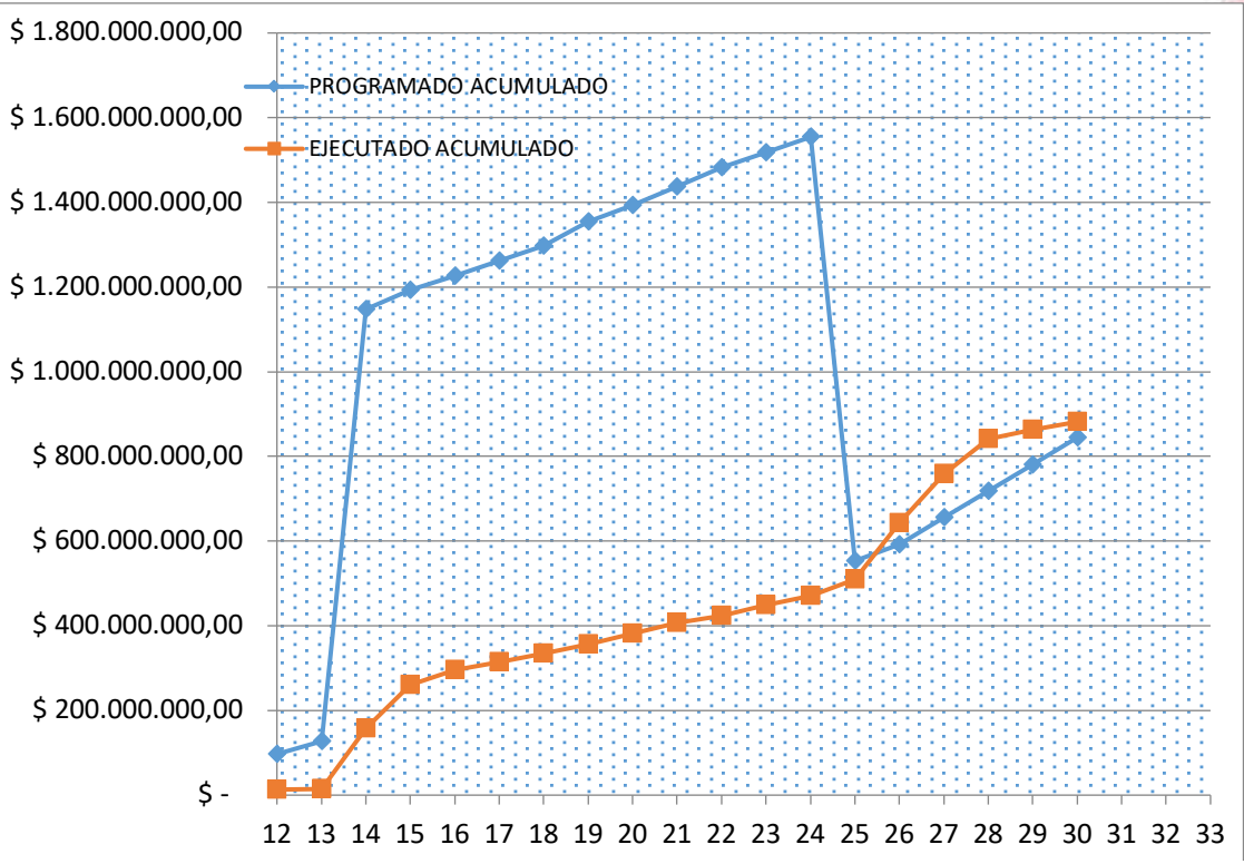
Ilustración 4 grafico de curva S de porcentajes de avance semanales, 2025. Fuente: Consorcio Interhospital PAC.
