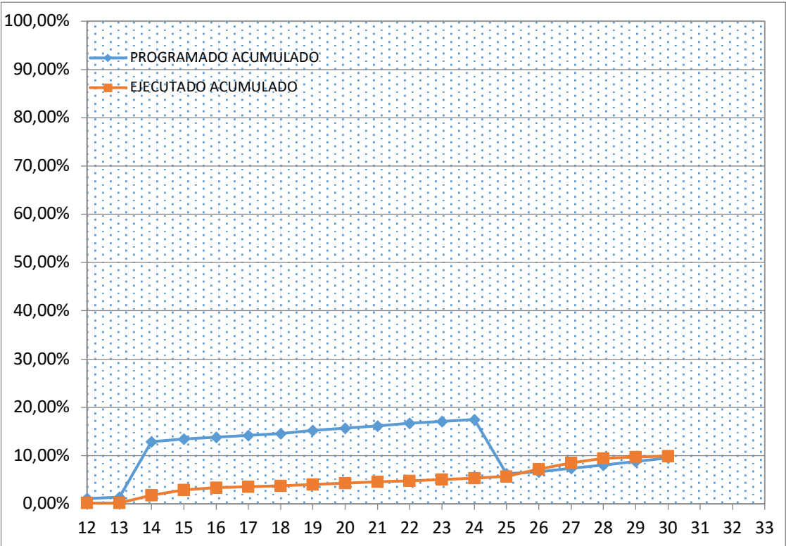
Ilustración 5 grafico de curva S de porcentajes de avance semanales, 2025. Fuente: Consorcio Interhospital PAC.
