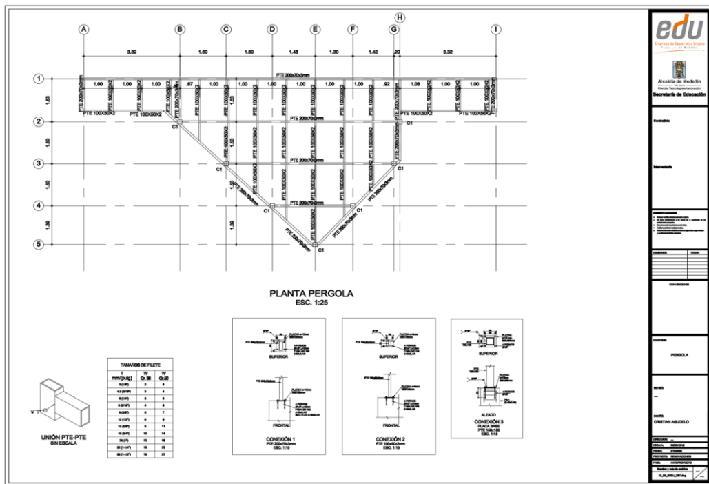
Ilustración 11. Planimetría diseño estructural de pérgola
