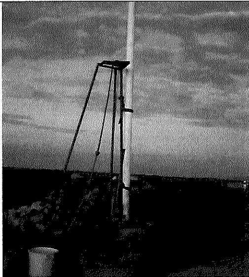
Suministro tubería 6"
