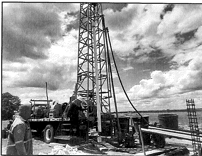
Imagen 3 Frente de trabajo libre de residuos, sin afectación A bosques (comunidad Puerto Lopez)
