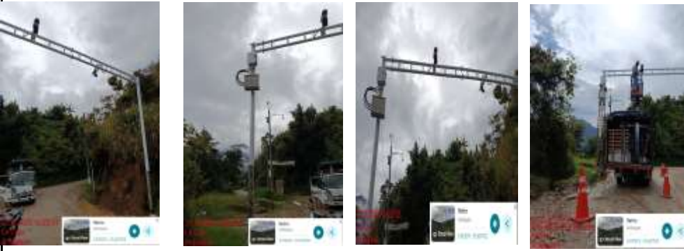
Suministro e instalación sistema LPR para dos sentidos viales, incluye sistema de comunicaciones y licenciamiento anual . UBICACIÓN: EL TABLERO
