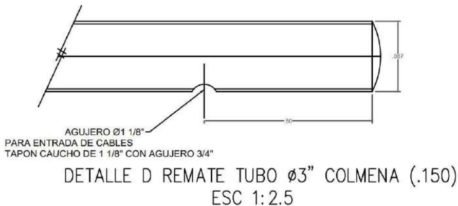
Figura 8. Detalle de remate de tubo de 3".
