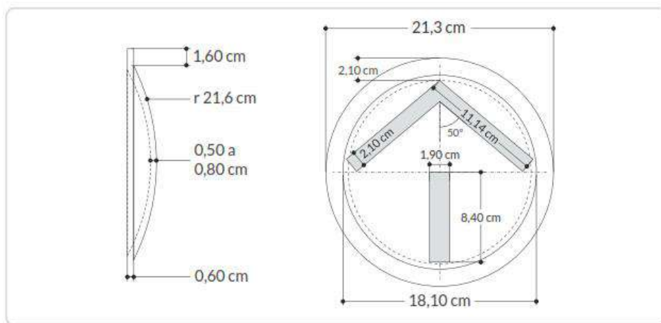
Figura 4-11. Dimensiones y configuración en flechas
