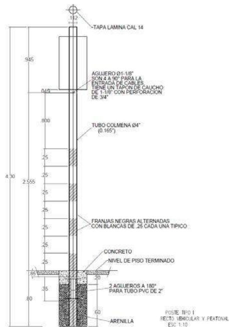
Figura 1. Detalle de poste recto de enterramiento directo.
