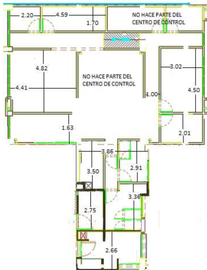
Esquema de centro de control
