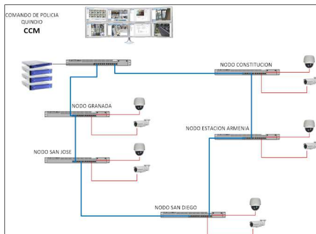
Gráfica de Topología de red cámaras CCTV
