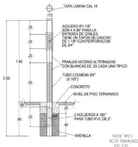
Figura 2. Detalle de poste recto de enterramiento directo para sonorizador.
