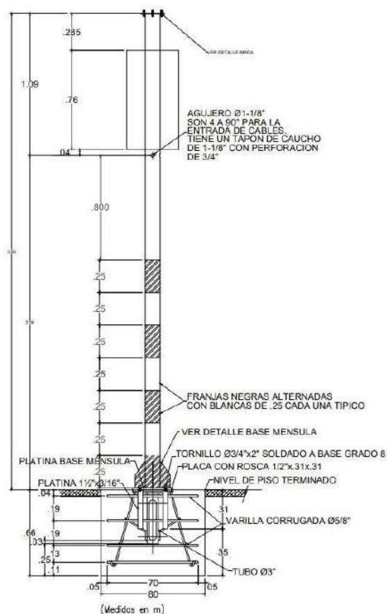
Figura 5. Detalle poste tipo III (Base platina y brida).
