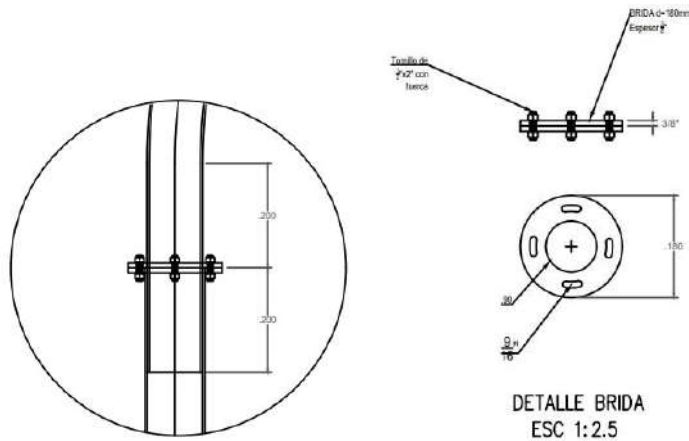
Figura 9. Detalle de brida de ménsula.
