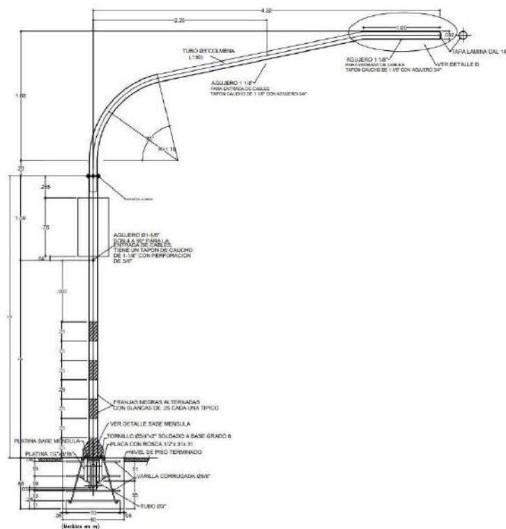
Figura 7. Detalle de poste tipo II con ménsula.
