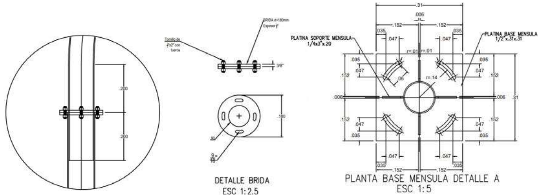
Figura 6. Detalle poste de base platina y brida.
