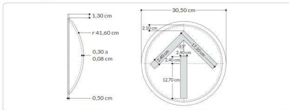
Figura 4-11. Dimensiones y configuración en flechas (continuación)
