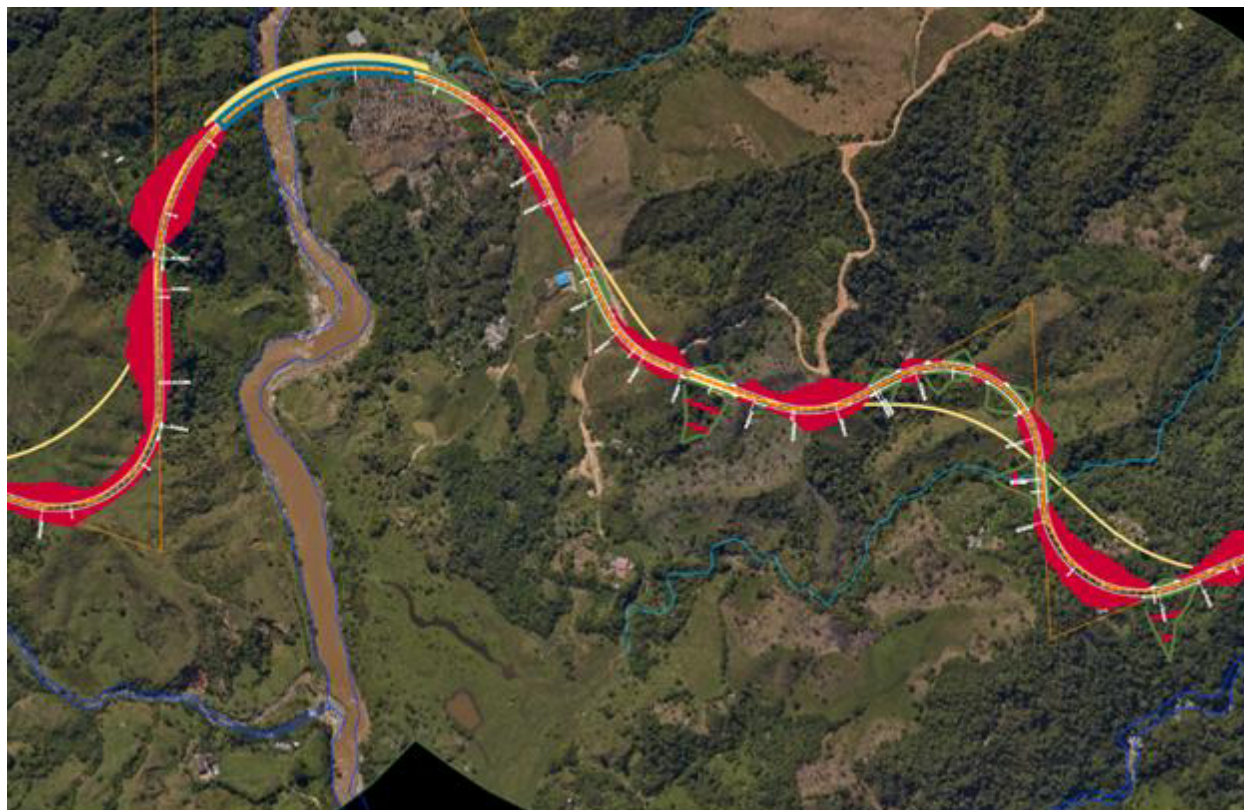
Ilustración 13. Revisión ponteadero Río Nare
