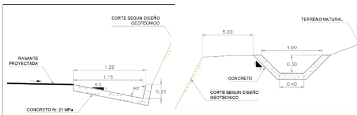
Ilustración 15. Predimensionamiento ODL
