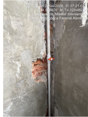
FOTO 2: Instalación de tubería de agua potable - Colegio Republica Federal Alemania
