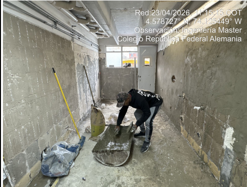
FOTO 1: Pañete de muros - Colegio Republica Federal Alemania
