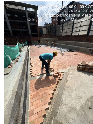
FOTO 2: Renovación de adoquín - Colegio Javier Matiz B
