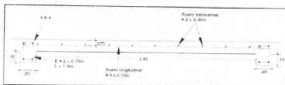
Ilustración 4. Detalle Viga.
