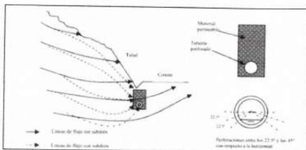
Ilustración 6. Esquema de dren. Fuente: PAVCO (2015).
