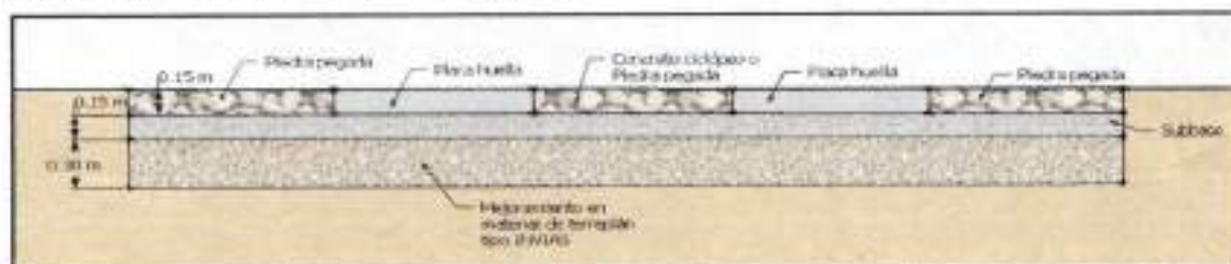
Ilustración 2. Estructura placa huella, Tramo N°02.
