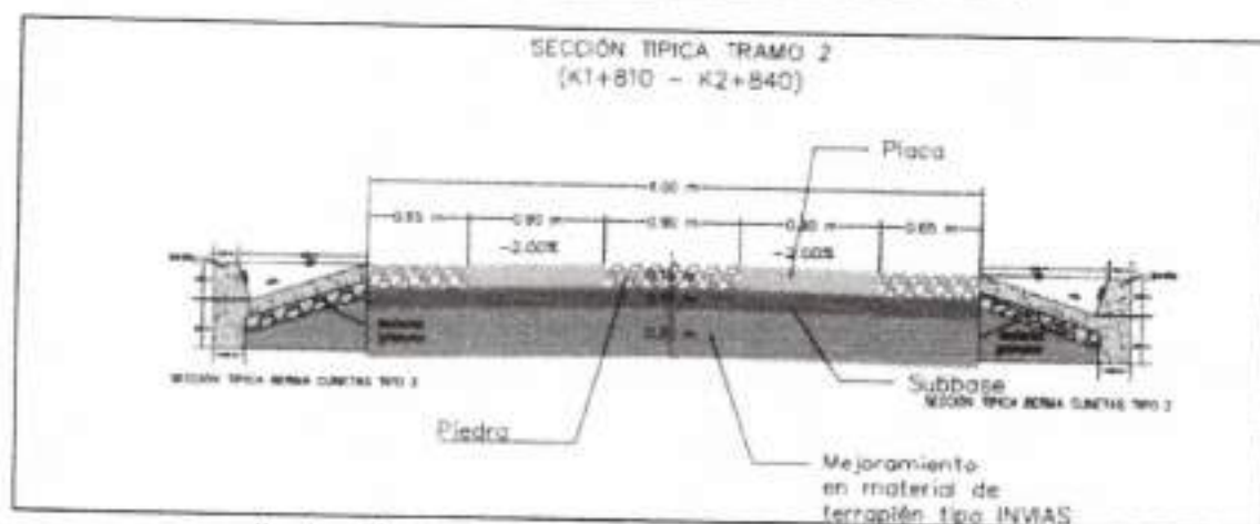
Ilustración 3. Estructura placa huella, Tramo N°02.
