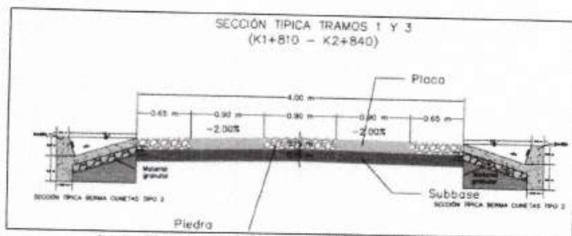
Ilustración 2. Estructura placa huella, Tramo N°01 y 03.
