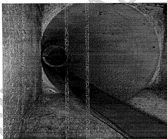
Vista Interna Estructura -- Entrada del Sistema a Estructura - 42" CR
