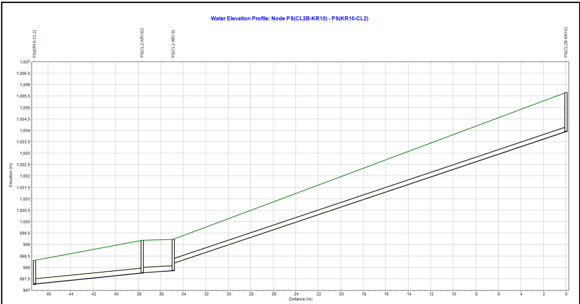
Figura 26. Perfil de tramo de alcantarillado sanitario con nivel de superficie de agua EDS #10 - Alternativa 1
