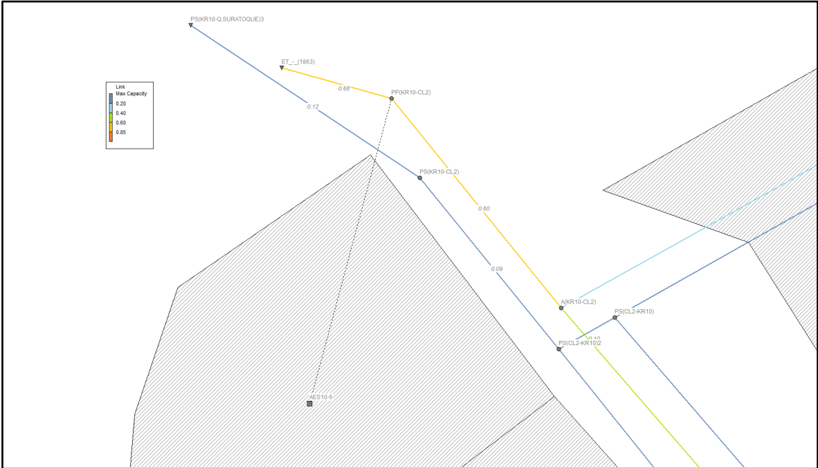
Figura 25. Esquema y capacidad en los tramos del modelo swmm EDS #10 - Alternativa 1
