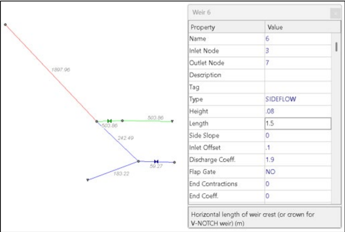
Figura 48. Esquema y capacidad en los tramos del modelo swmm EDS #14 - Alternativa 1
