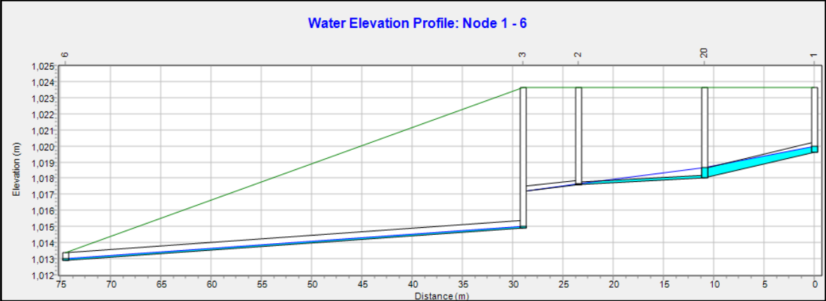
Figura 15. Perfil de tramo de alcantarillado con nivel de superficie de agua_2 EDS #3 – Alternativa 2
