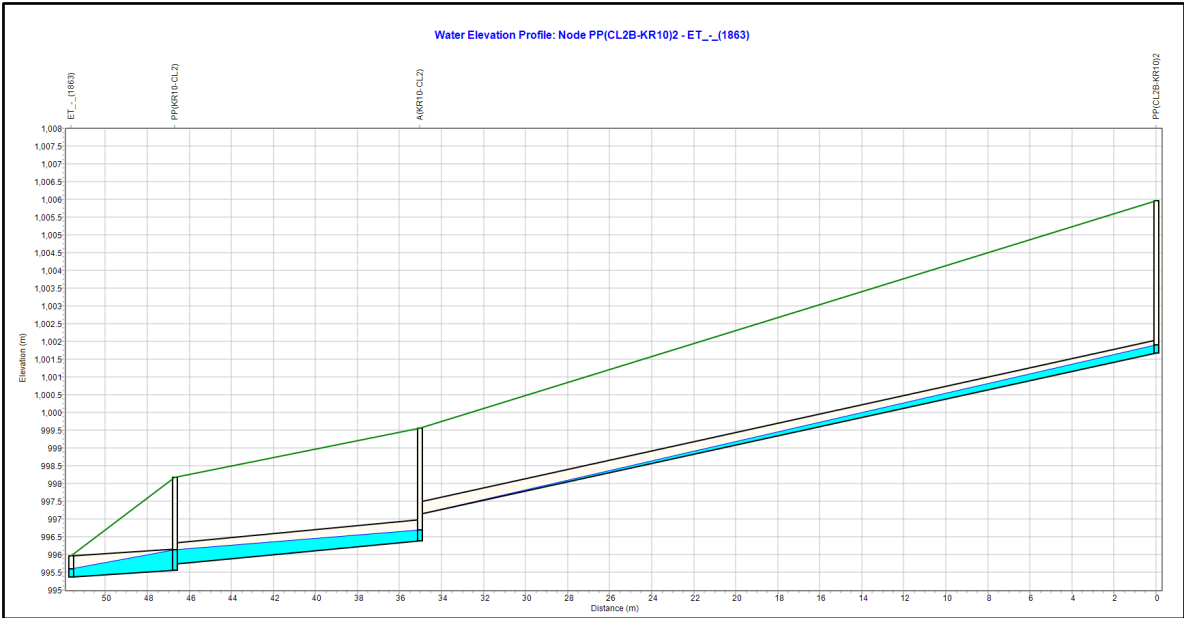
Figura 30. Perfil de tramo de alcantarillado pluvial con nivel de superficie de agua EDS #10 - Alternativa 2
