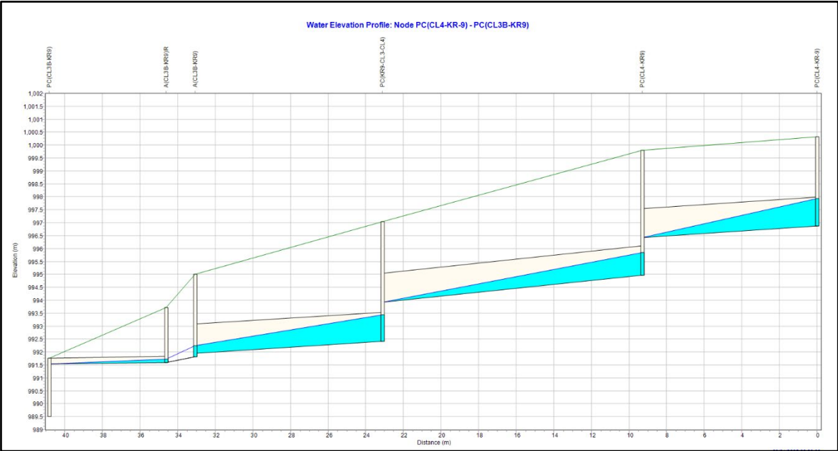
Figura 35. Perfil de tramo de alcantarillado con nivel de superficie de agua EDS #11 - Alternativa 2
