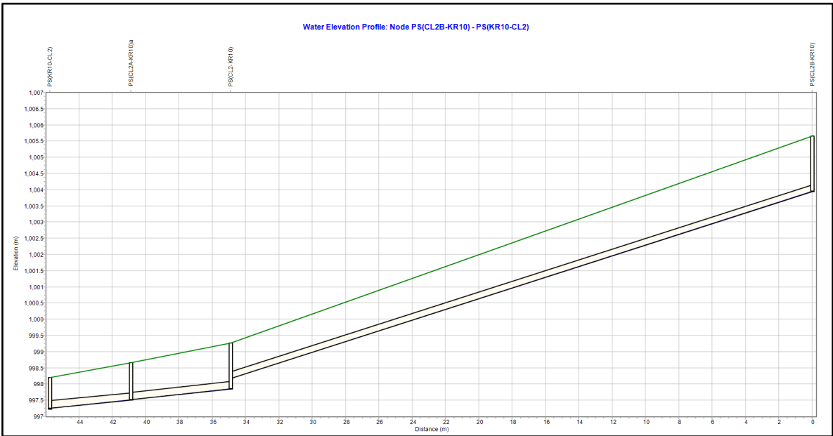
Figura 29. Perfil de tramo de alcantarillado sanitario con nivel de superficie de agua EDS #10 – Alternativa 2
