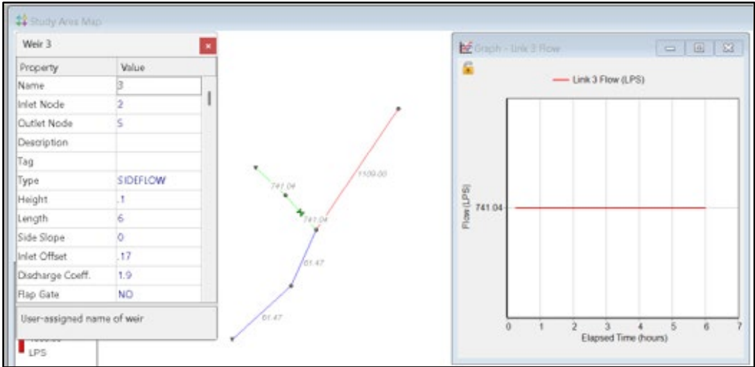
Figura 43. Esquema y capacidad en los tramos del modelo swmm EDS #13 - Alternativa 1
