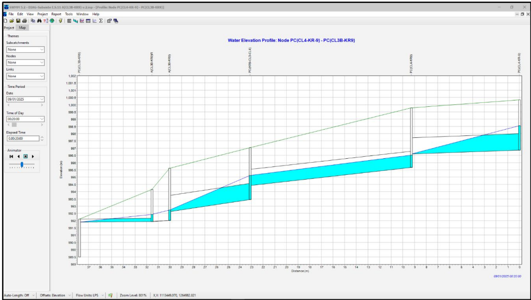
Figura 32. Perfil de tramo de alcantarillado con nivel de superficie de agua EDS #11
