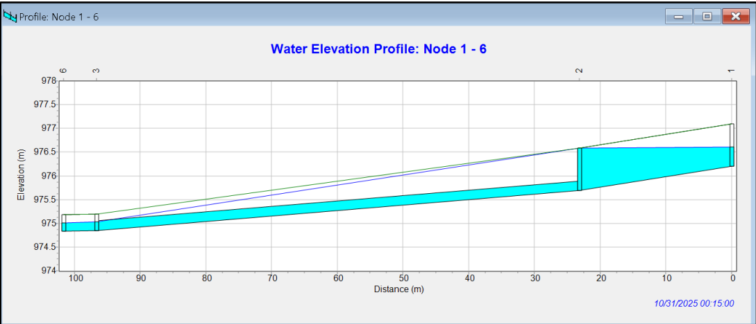
Figura 44. Perfil de tramo de alcantarillado sanitario con nivel de superficie de agua EDS #13 - Alternativa 1
