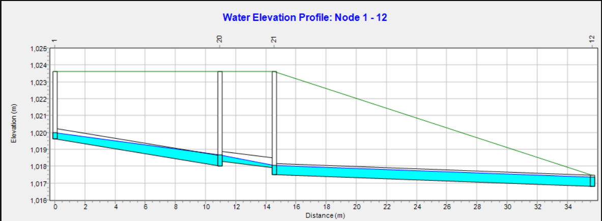
Figura 14. Perfil de tramo de alcantarillado con nivel de superficie de agua_1 EDS #3 – Alternativa 2
