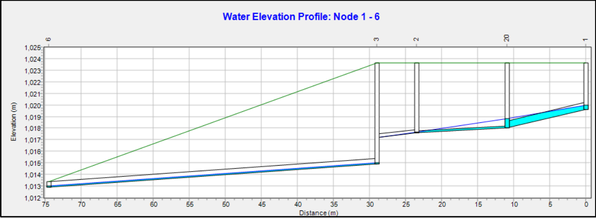
Figura 13. Perfil de tramo de alcantarillado con nivel de superficie de agua_2 EDS #3 – Alternativa 1
