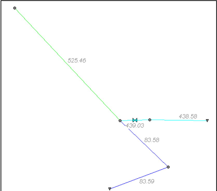
Figura 5. Sistema propuesto contracción en salida sanitaria - modelo swmm EDS #1 - Alternativa 1
