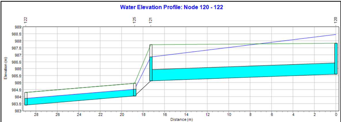
Figura 38. Perfil del tramo de alcantarillado con nivel de superficie de agua_2 EDS #12
