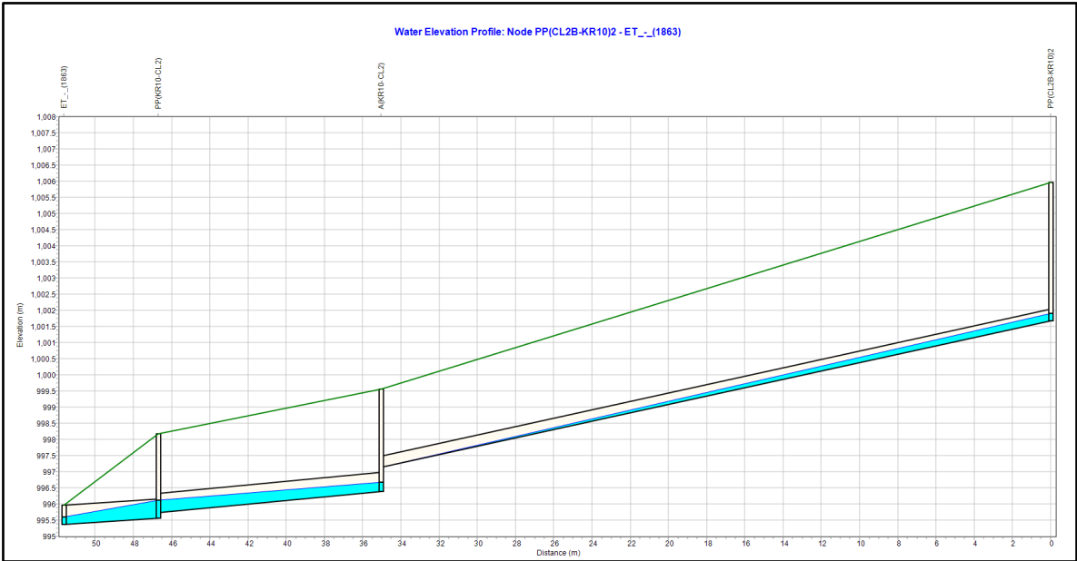
Figura 27. Perfil de tramo de alcantarillado pluvial con nivel de superficie de agua EDS #10 - Alternativa 1
