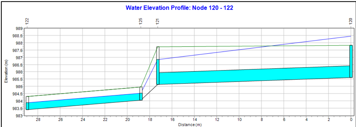
Figura 8. Perfil de tramo de alcantarillado con nivel de superficie de agua_2 EDS #3
