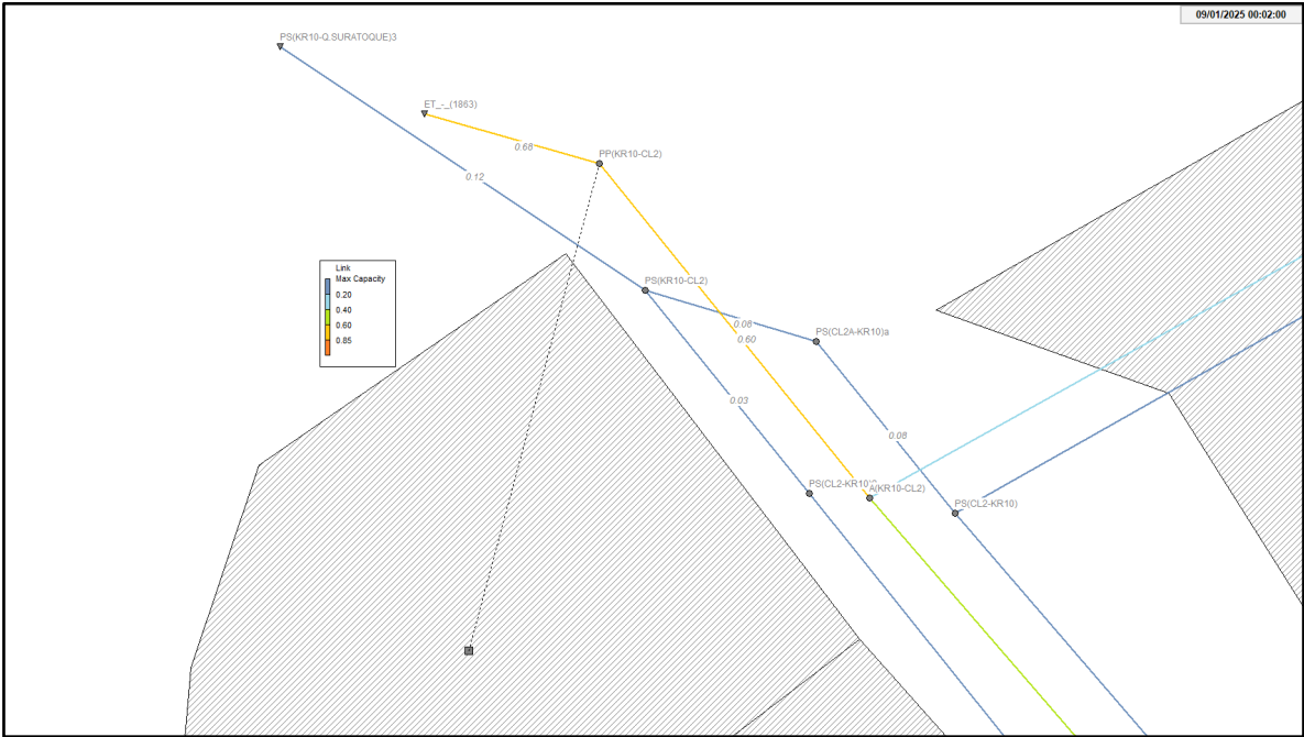
Figura 28. Esquema y capacidad en los tramos del modelo swmm EDS #10 - Alternativa 2
