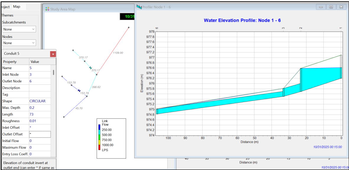
Figura 46. Perfil de tramo de alcantarillado sanitario con nivel de superficie de agua EDS #13 - Alternativa 2
