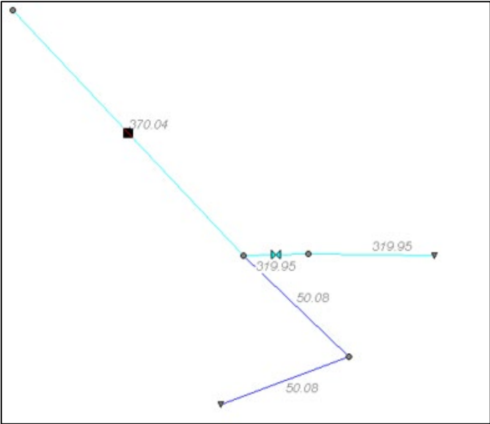
Figura 6. Sistema propuesto contracción en salida sanitaria - modelo swmm EDS #1 - Alternativa 2
