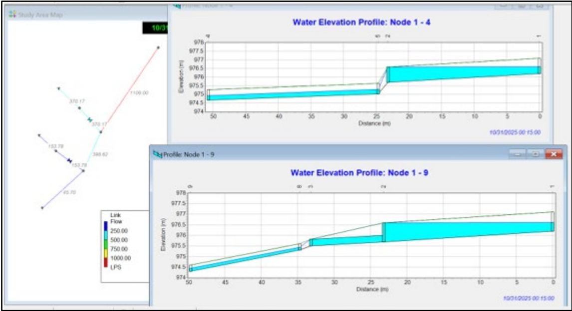
Figura 47. Perfil de tramo de alcantarillado pluvial con nivel de superficie de agua EDS #13 - Alternativa 2
