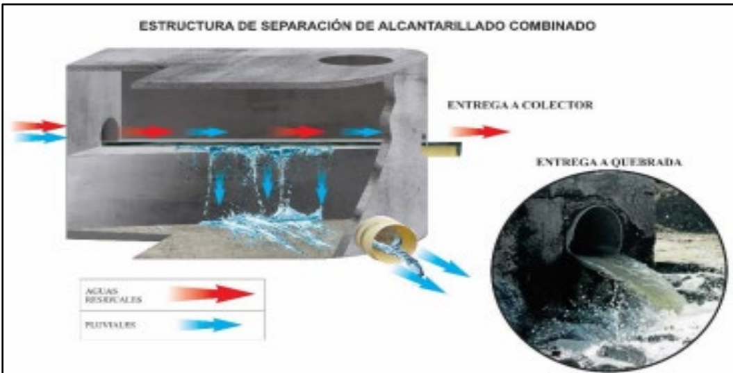
Figura 1. Estructura de Separación Típica del Alcantarillado Combinado
