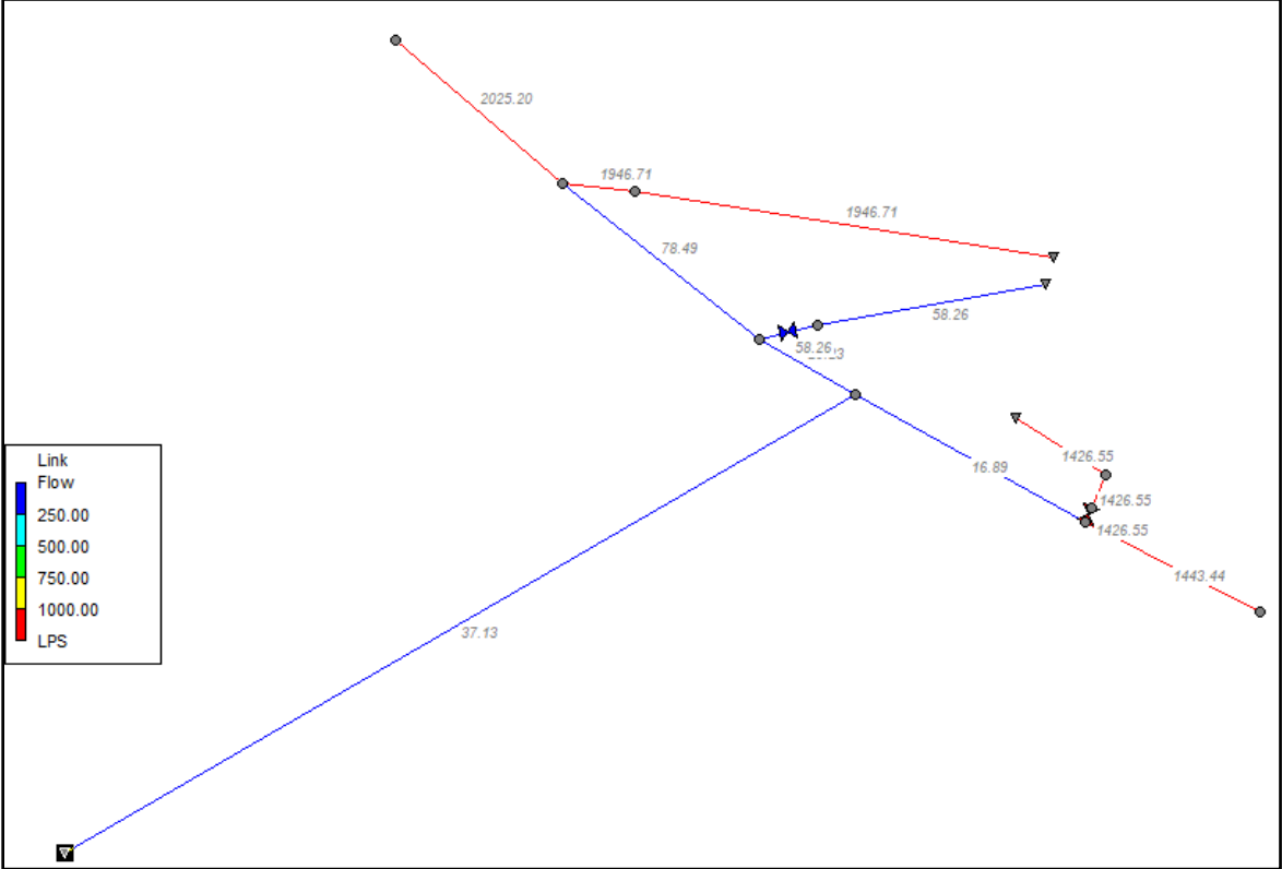
Figura 16. Esquema y caudales del modelo swmm_1 EDS #3 - Alternativa 2
