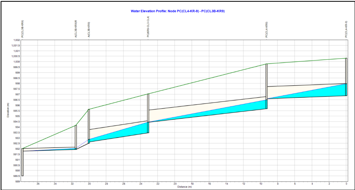
Figura 34. Perfil de tramo de alcantarillado con nivel de superficie de agua EDS #11 - Alternativa 1
