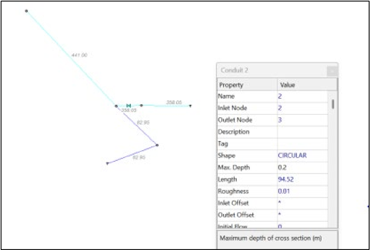
Figura 19. Sistema propuesto contracción en salida sanitaria - modelo swmm EDS #4 - Alternativa 1
