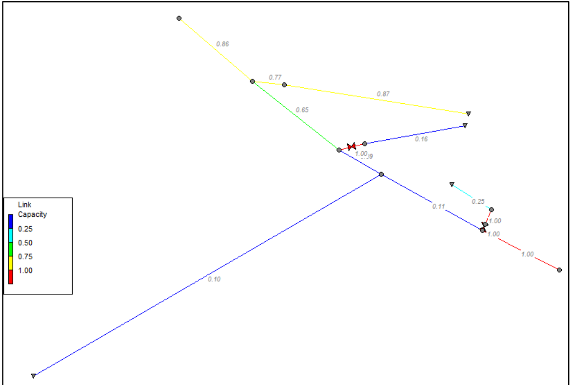
Figura 11. Esquema y caudales del modelo swmm_3 EDS #3 - Alternativa 1
