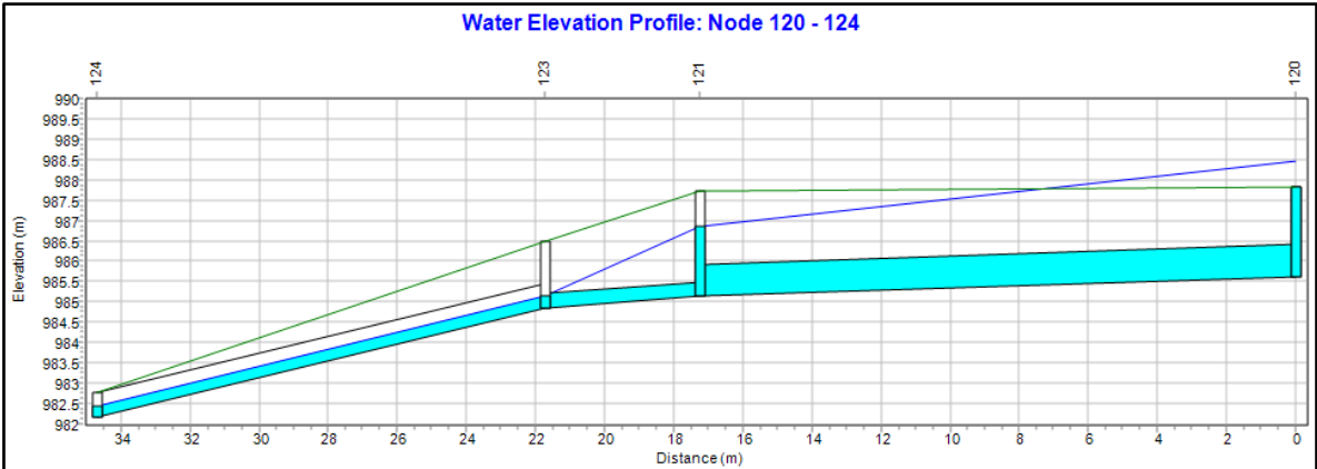
Figura 37. Perfil del tramo de alcantarillado con nivel de superficie de agua_1 EDS #12
