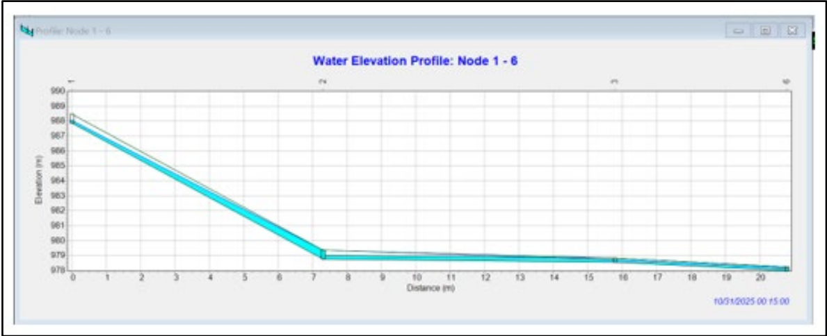
Figura 52. Perfil de tramo de alcantarillado sanitario con nivel de superficie de agua EDS #14 - Alternativa 2
