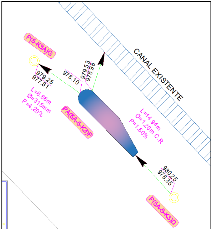
Figura 54. Planta General de la Estructura de separación #15
