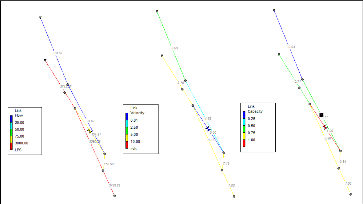
Figura 42. Esquema y caudales del modelo swmm EDS #12 - Alternativa 2
