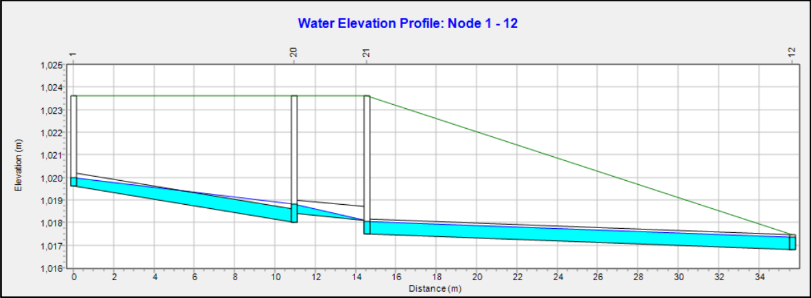
Figura 12. Perfil de tramo de alcantarillado con nivel de superficie de agua_1 EDS #3 – Alternativa 1
