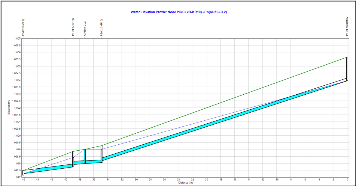
Figura 24. Perfil de tramo de alcantarillado sanitario con nivel de superficie de agua - EDS #10
