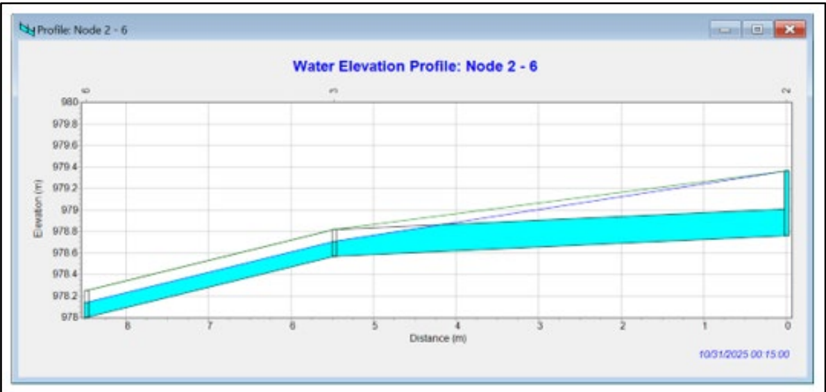
Figura 50. Perfil de tramo de alcantarillado pluvial con nivel de superficie de agua EDS #14 - Alternativa 1
