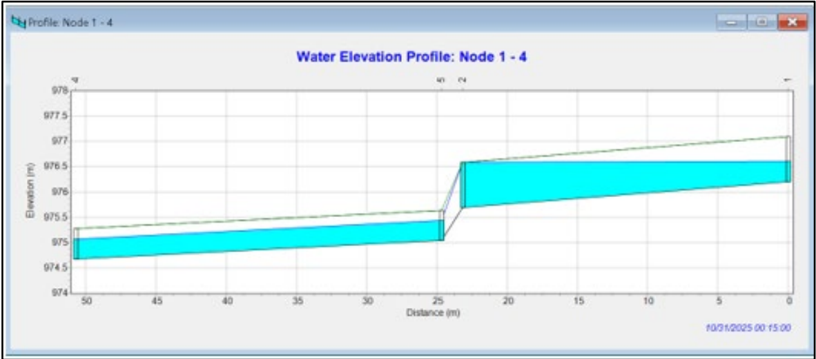
Figura 45. Perfil de tramo de alcantarillado pluvial con nivel de superficie de agua EDS #13 - Alternativa 1
