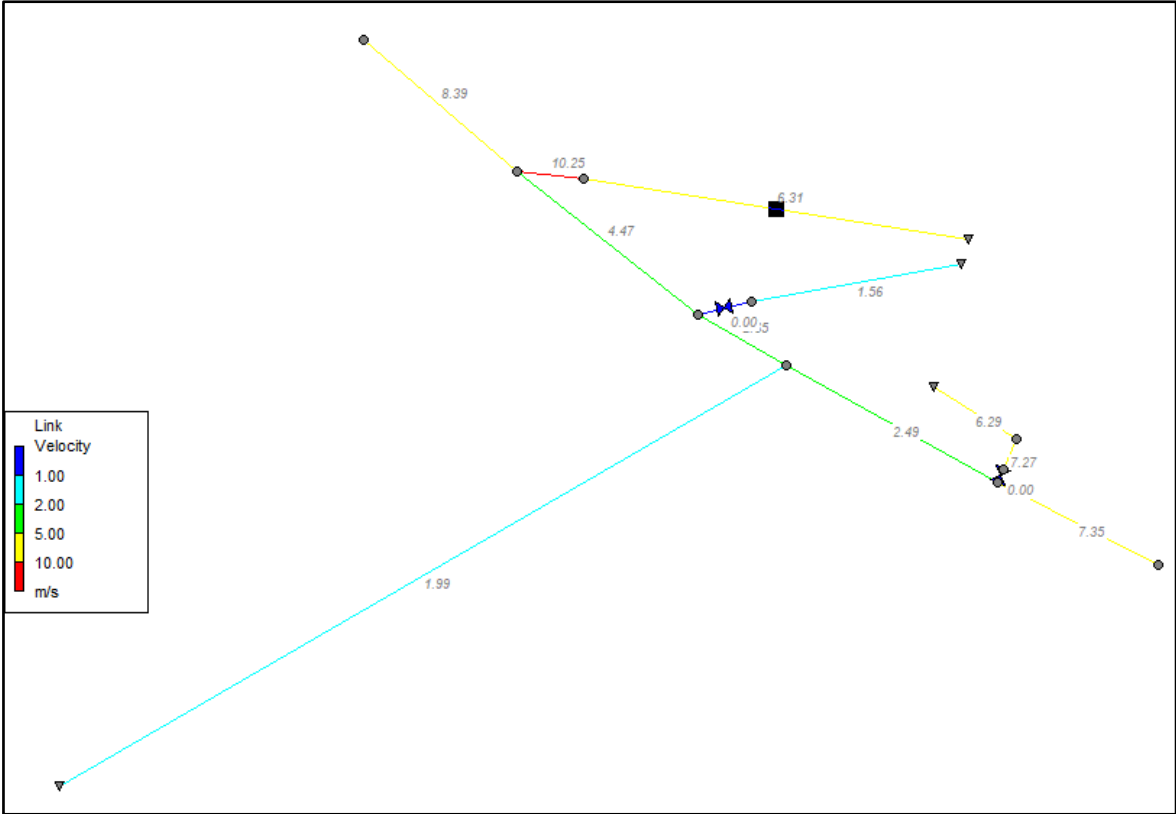
Figura 17. Esquema y caudales del modelo swmm_2 EDS #3 - Alternativa 2
