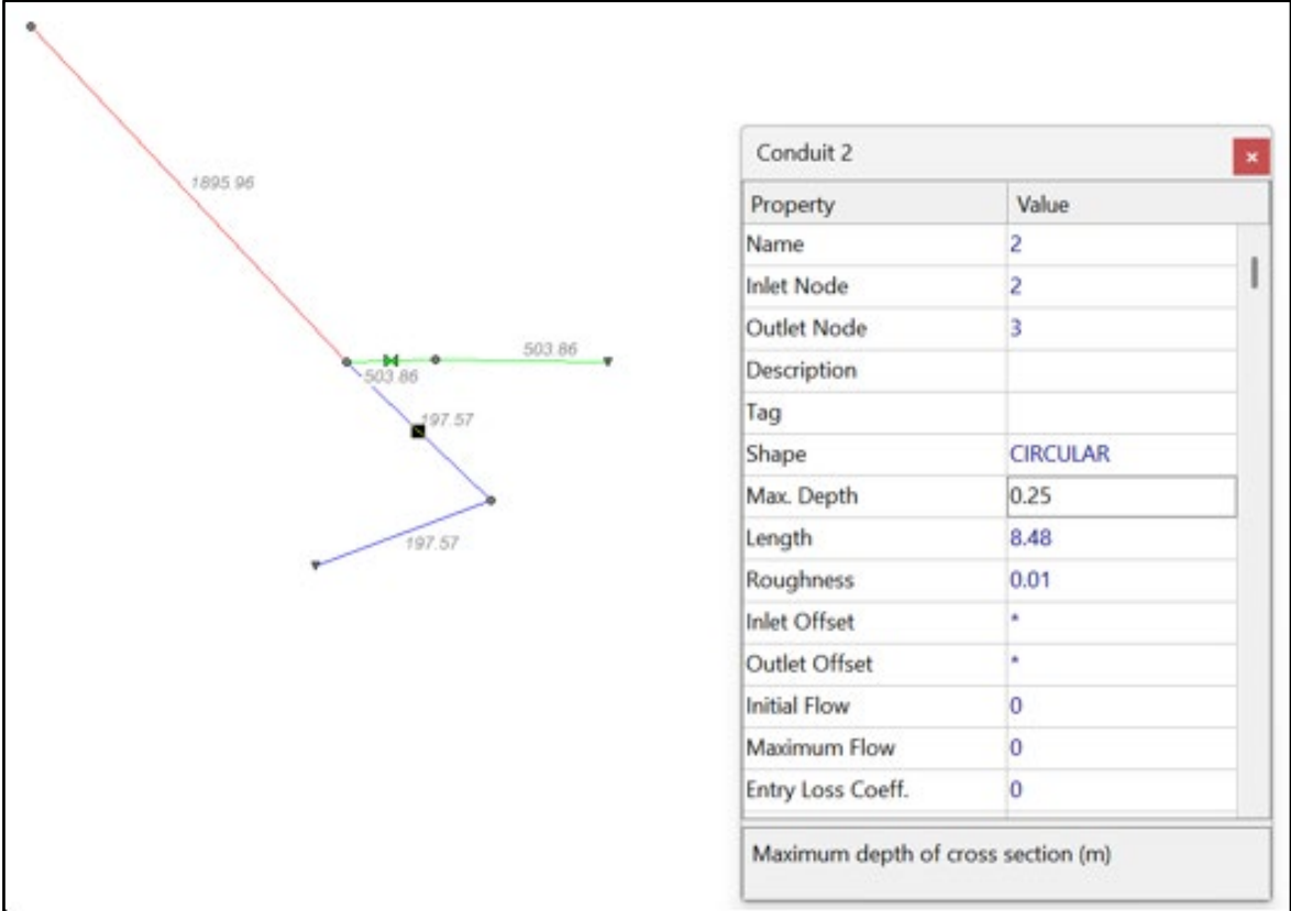
Figura 51. Esquema y capacidad en los tramos del modelo swmm EDS #14 - Alternativa 2
