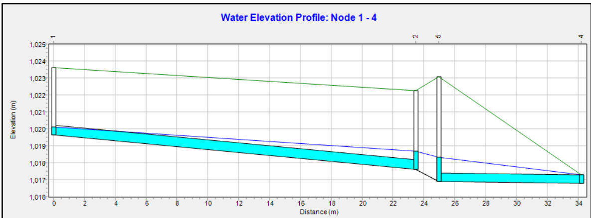
Figura 7. Perfil del tramo de alcantarillado con nivel de superficie de agua_1 EDS #3
