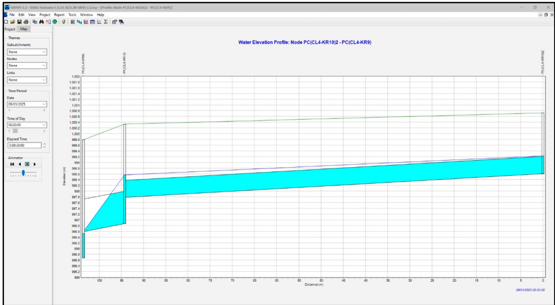
Figura 31. Perfil del tramo de alcantarillado con nivel de superficie de agua-EDS #11
