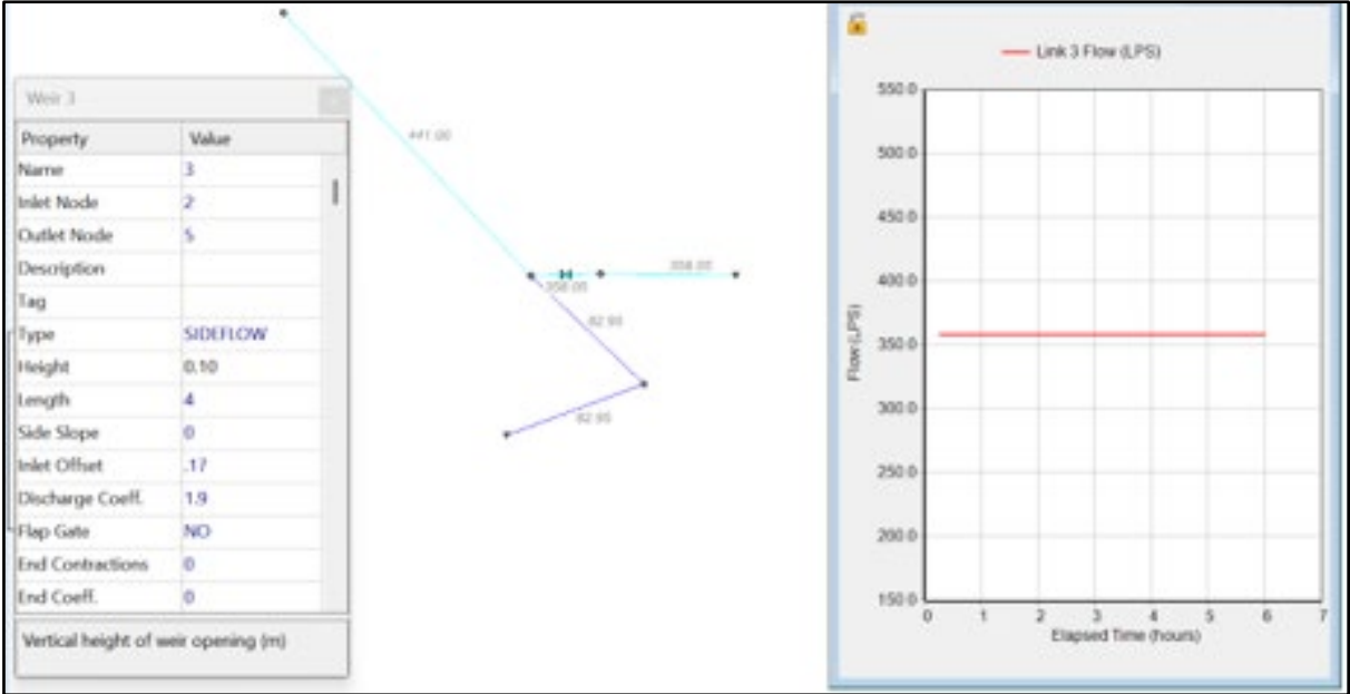
Figura 20. Perfil sanitario del sistema propuesto - modelo swmm EDS #4 - Alternativa 1
