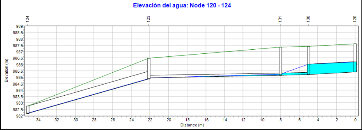
Figura 41. Perfil de tramo de alcantarillado sanitario con nivel de superficie de agua EDS #12 - Alternativa 2
