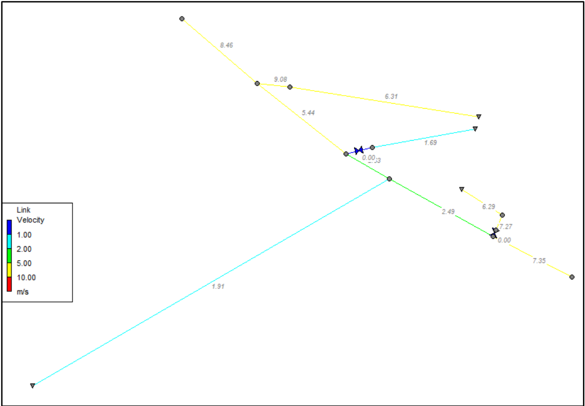
Figura 10. Esquema y caudales del modelo swmm_2 EDS #3 – Alternativa 1
