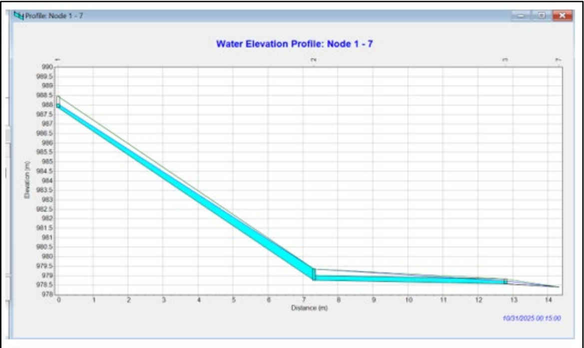
Figura 49. Perfil de tramo de alcantarillado sanitario con nivel de superficie de agua EDS #14 - Alternativa 1
