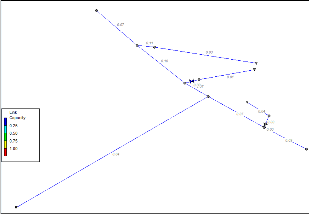
Figura 18. Esquema y caudales del modelo swmm_3 EDS #3 - Alternativa 2
