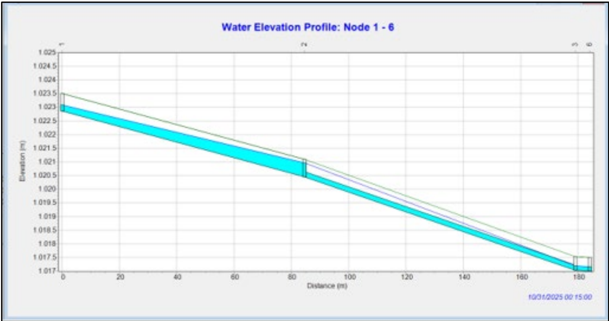
Figura 21. Perfil de tramo de alcantarillado pluvial con nivel de superficie de agua EDS #4 - Alternativa 1
