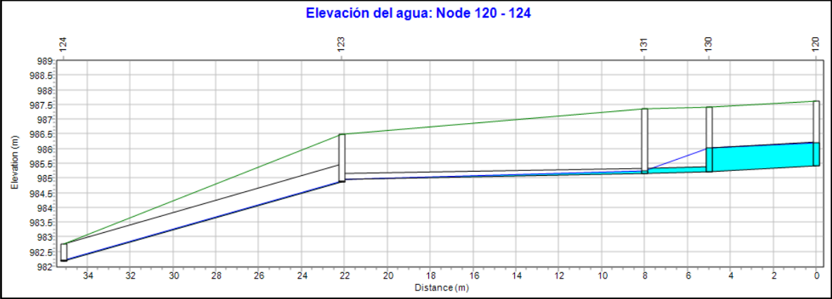
Figura 40. Perfil de tramo de alcantarillado sanitario con nivel de superficie de agua EDS #12 - Alternativa 1
