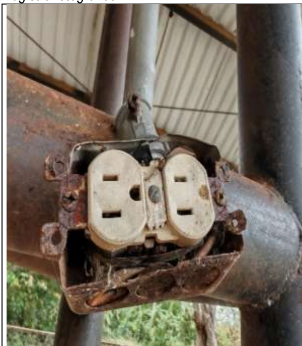
Foto 1: Estado Inicial punto eléctrico
