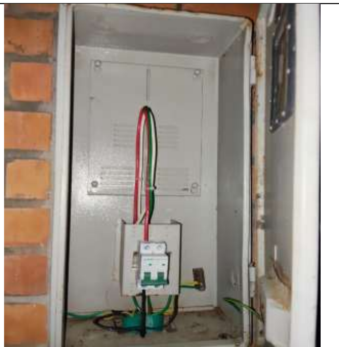
Foto 2: cable 8 AWG cobre de color rojo instalado
