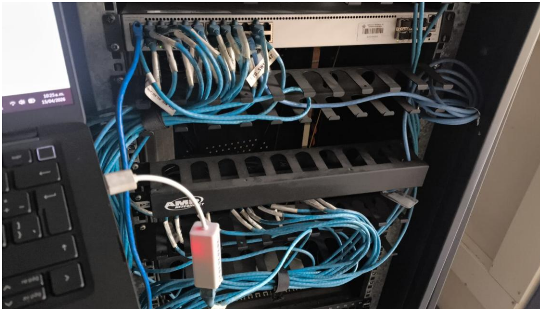
Verificación de VLAN de la sede de meissen.
