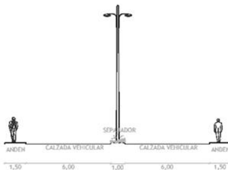
SECCION TRANSVERSAL VIA V2
