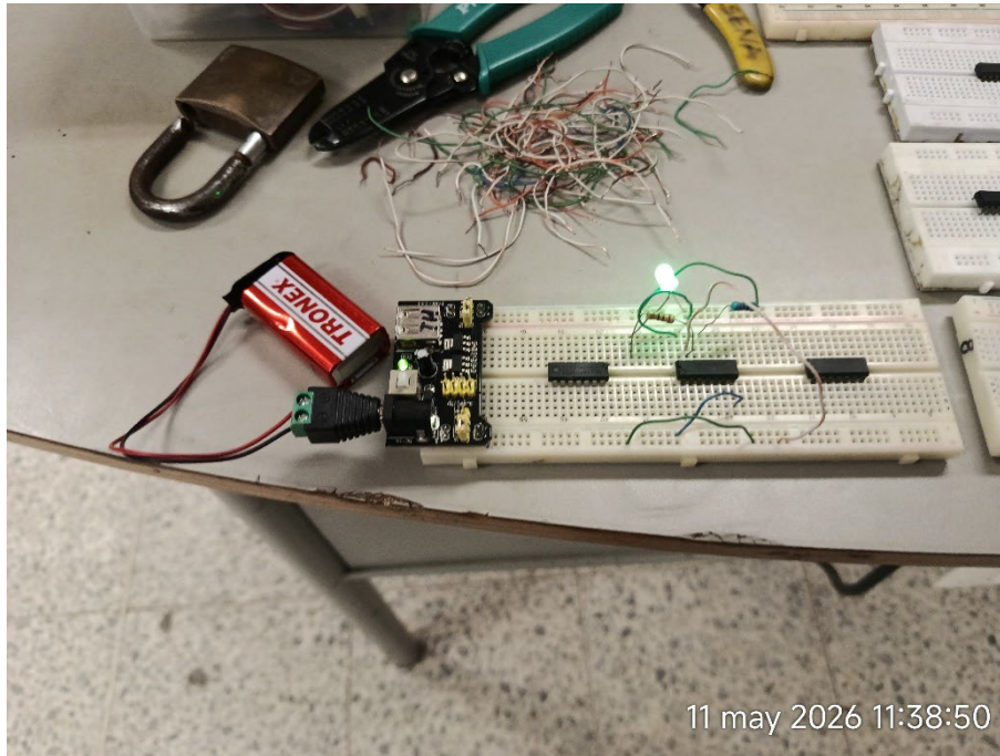
Figura 3. Actividades de electrónica digital fichas 3151761 3151771 CEMM
