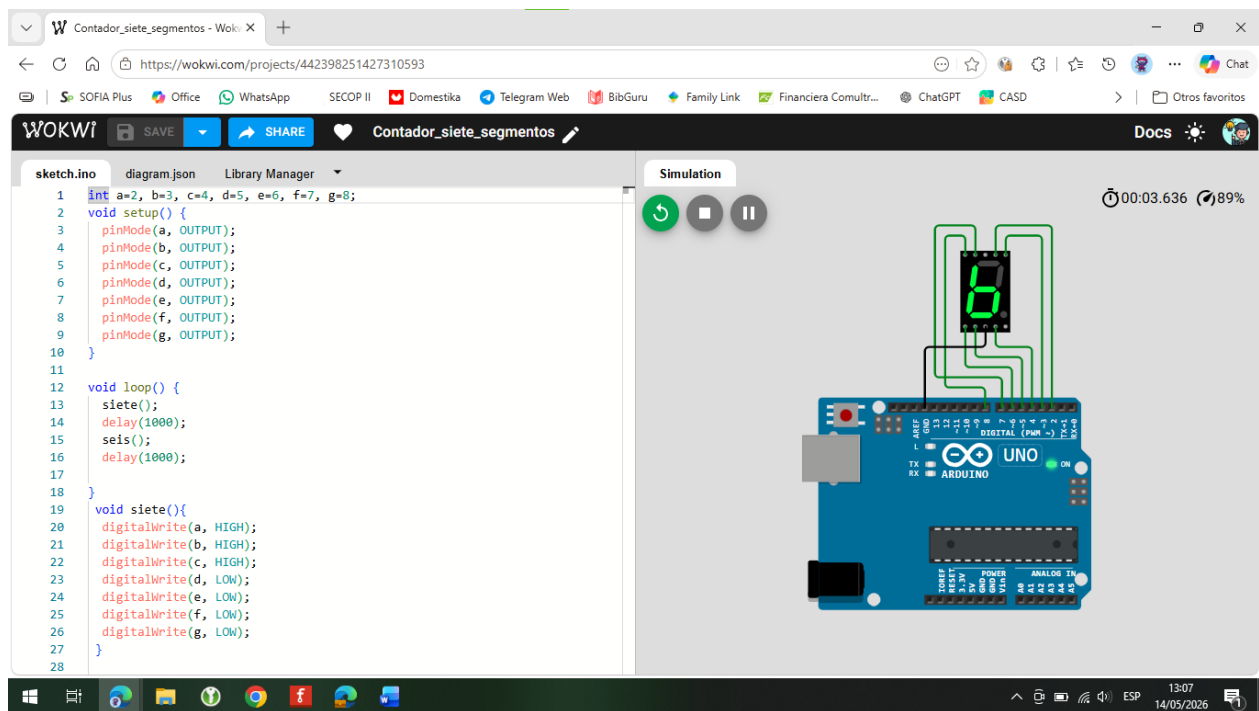
Figura 2. Actividad simulador Wokwi ficha 3151872 ITS1
