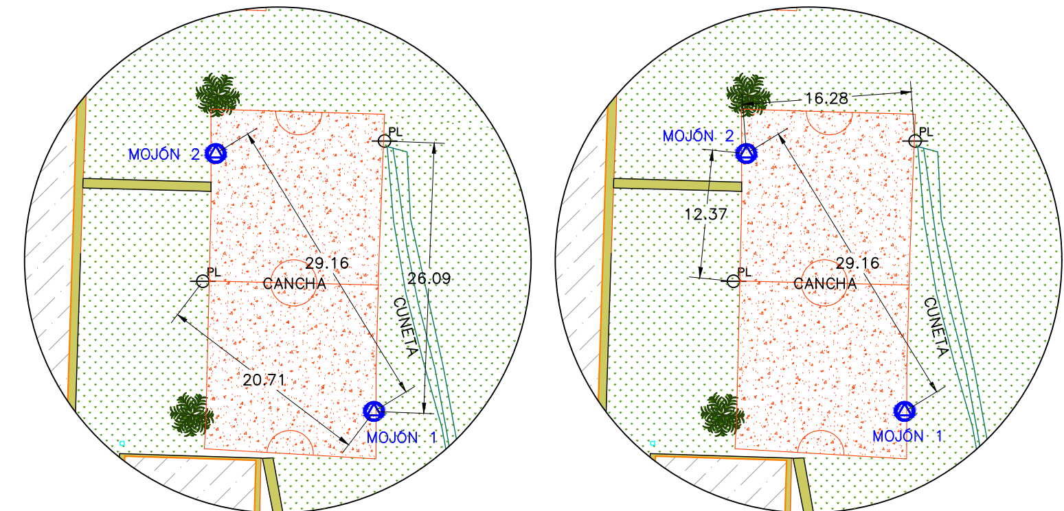
REFERENCIA DE MOJONES ESCALA: 1:500
