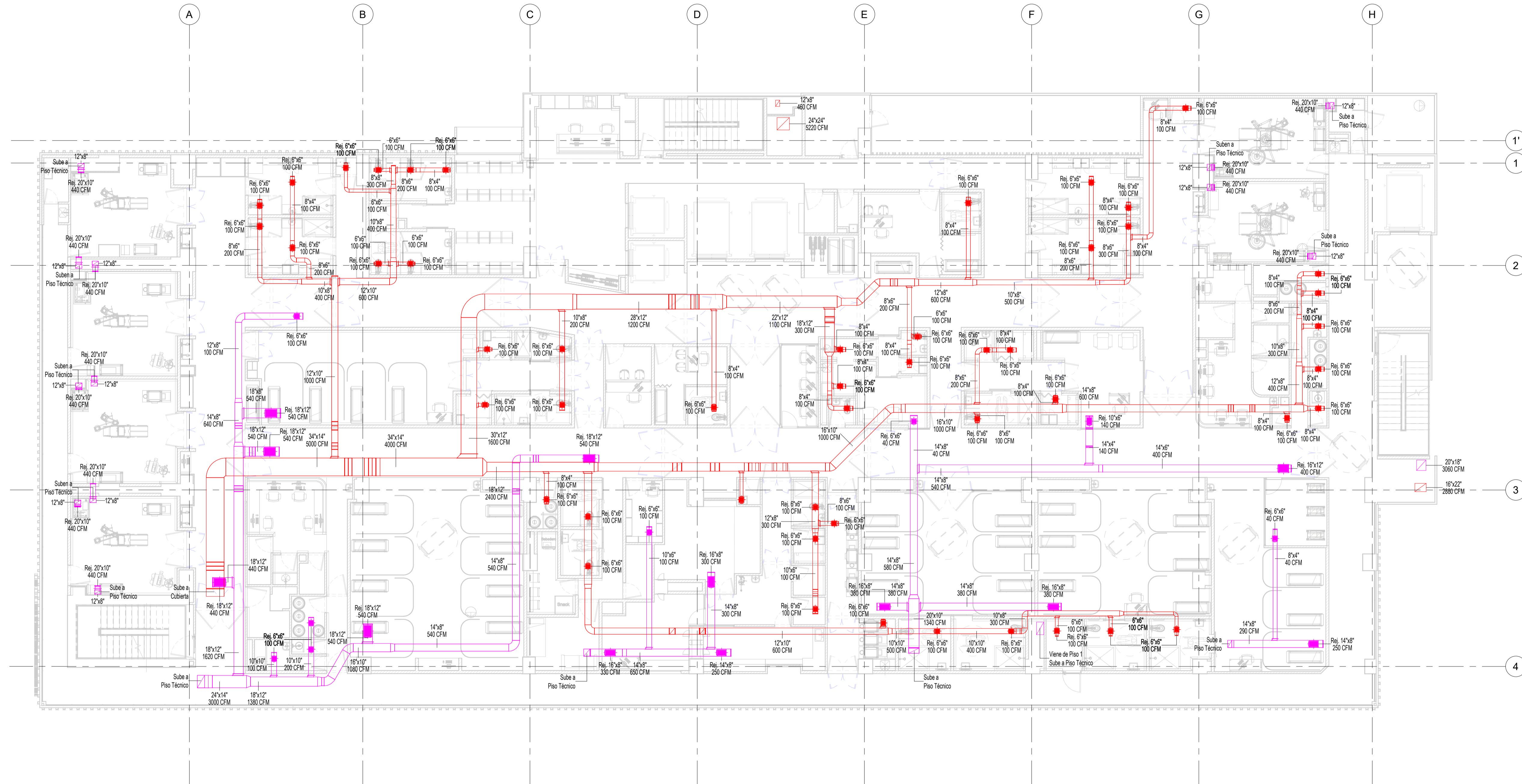
03. PLANTA DE VENTILACIÓN MECÁNICA - EXTRACCIÓN DE AIRE PISO 2 1 : 100
