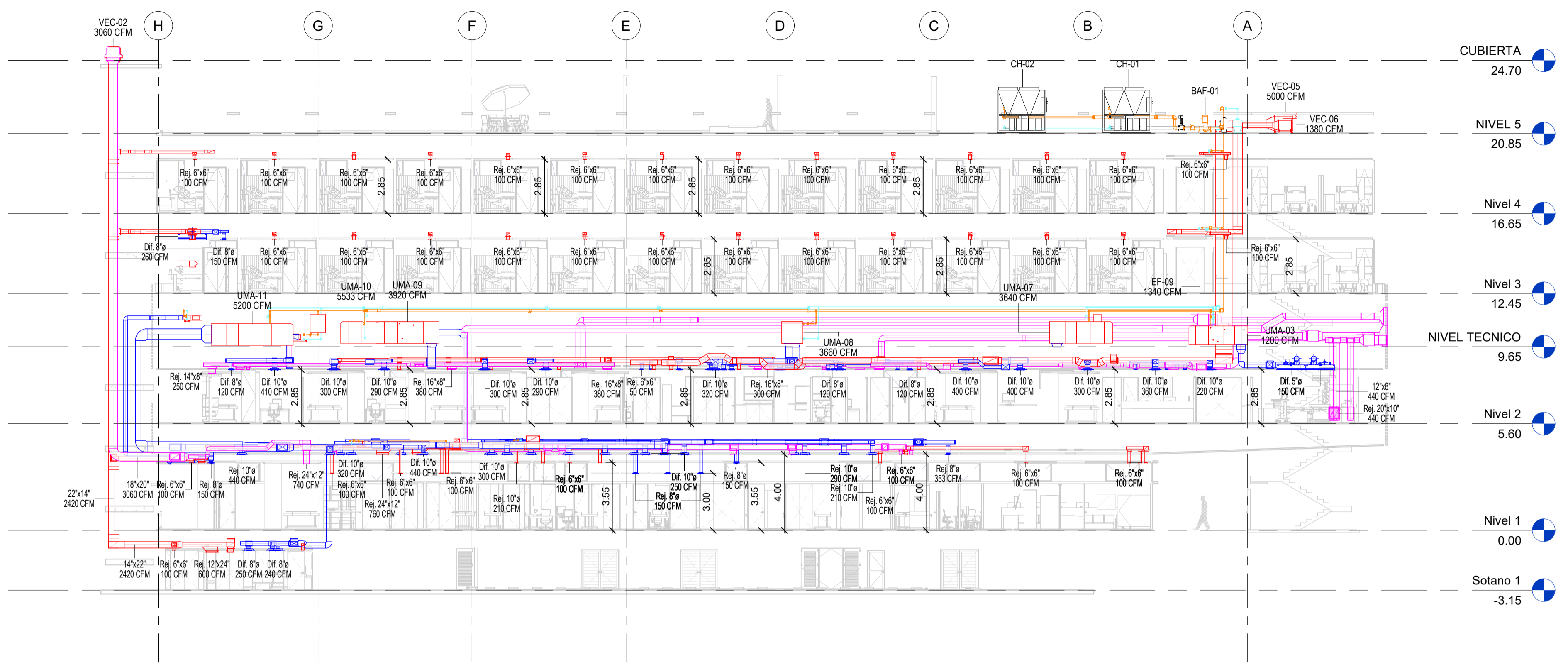
1 CORTE LONGITUDINAL A-A 1:150
