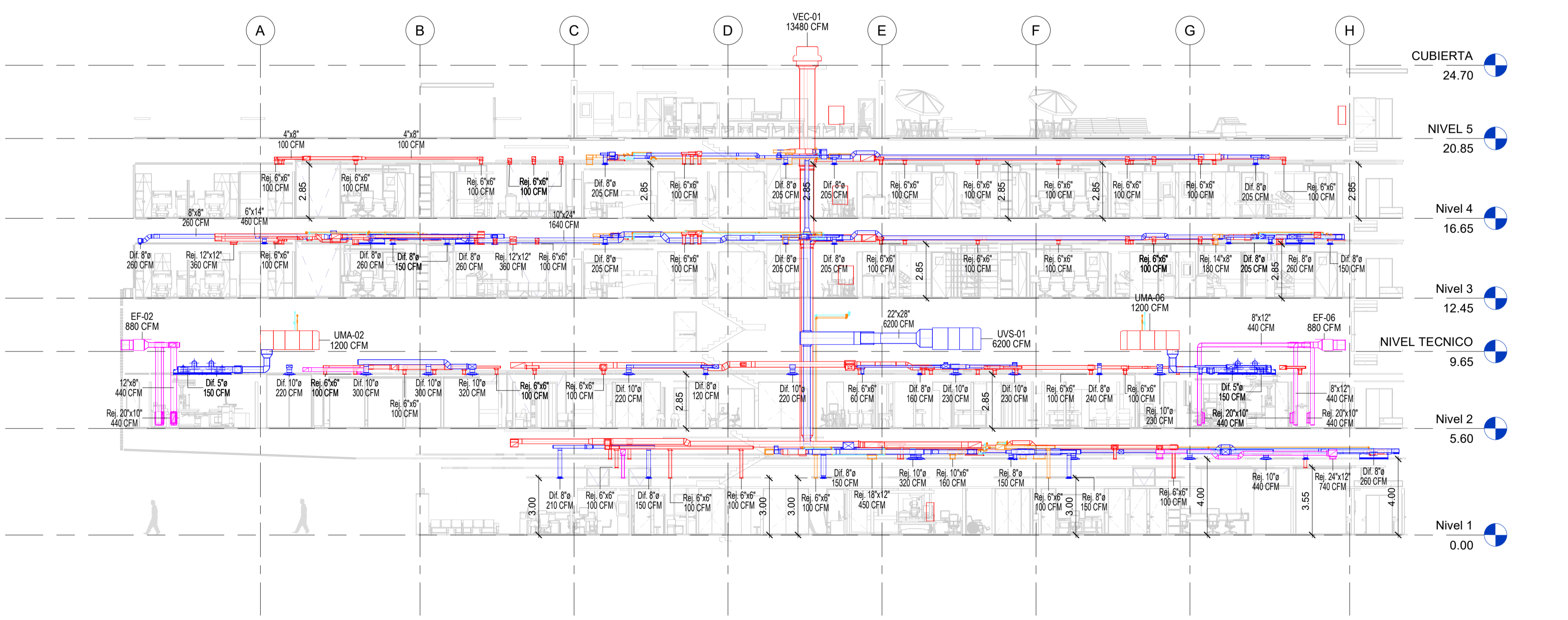
2 CORTE LONGITUDINAL B-B 1:150
