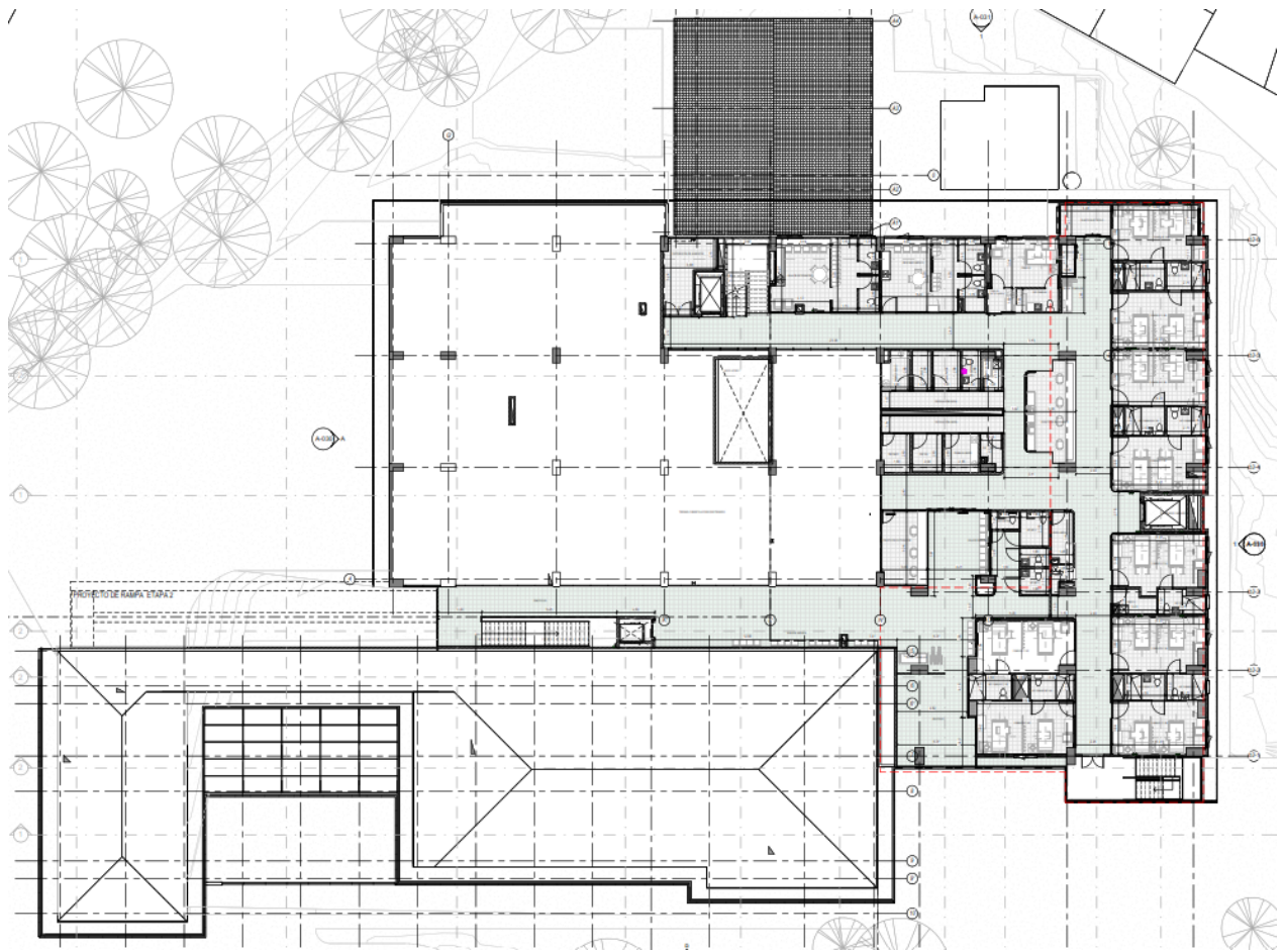
Planta nivel -1
