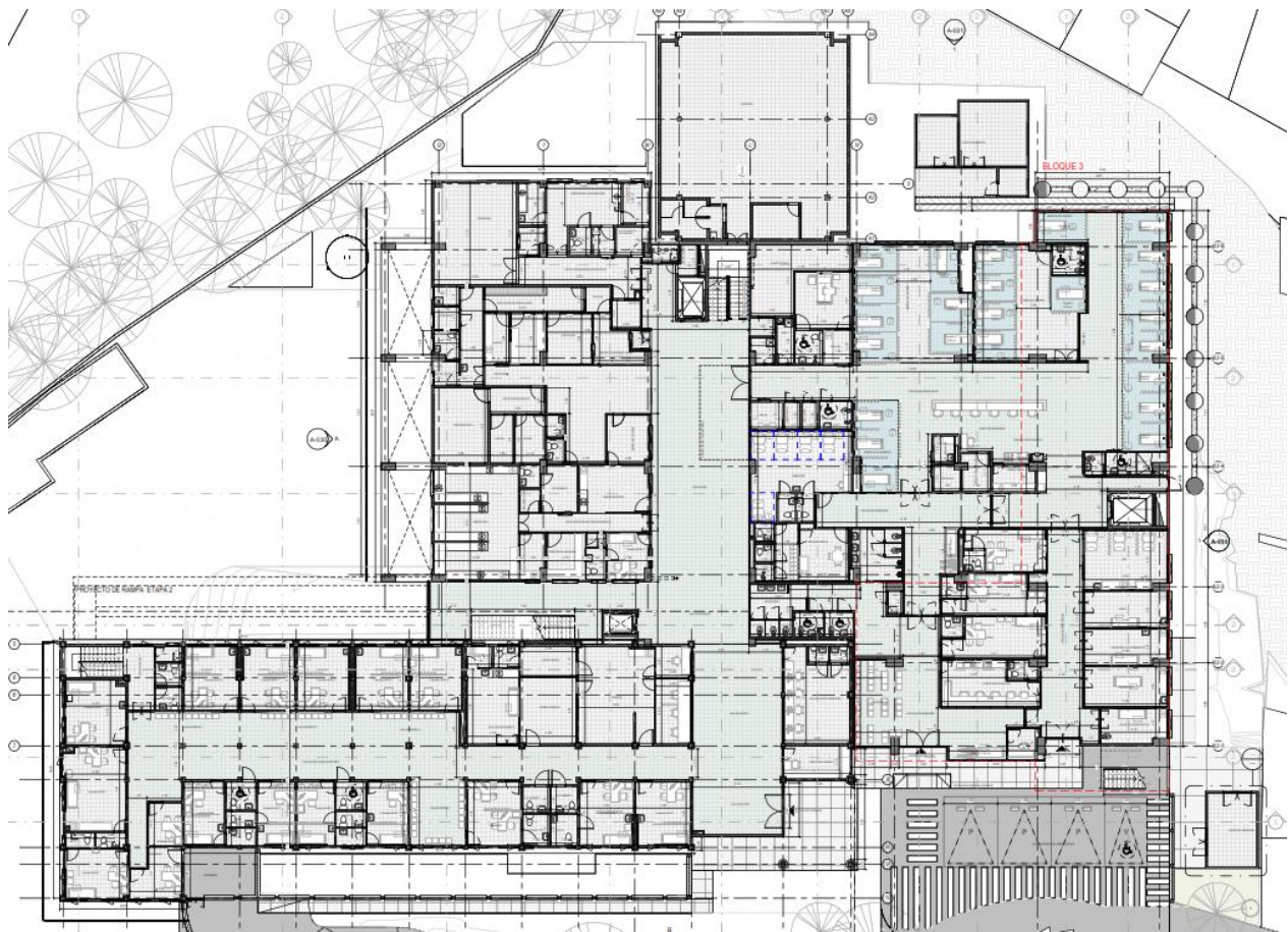
Planta Nivel 2
