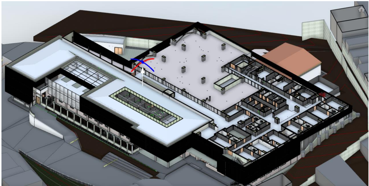
Isométrico nivel 2
