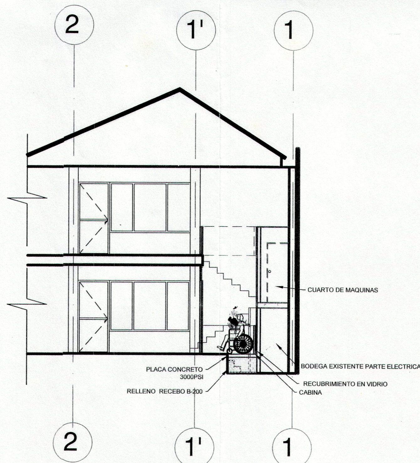
Corte R - R'
