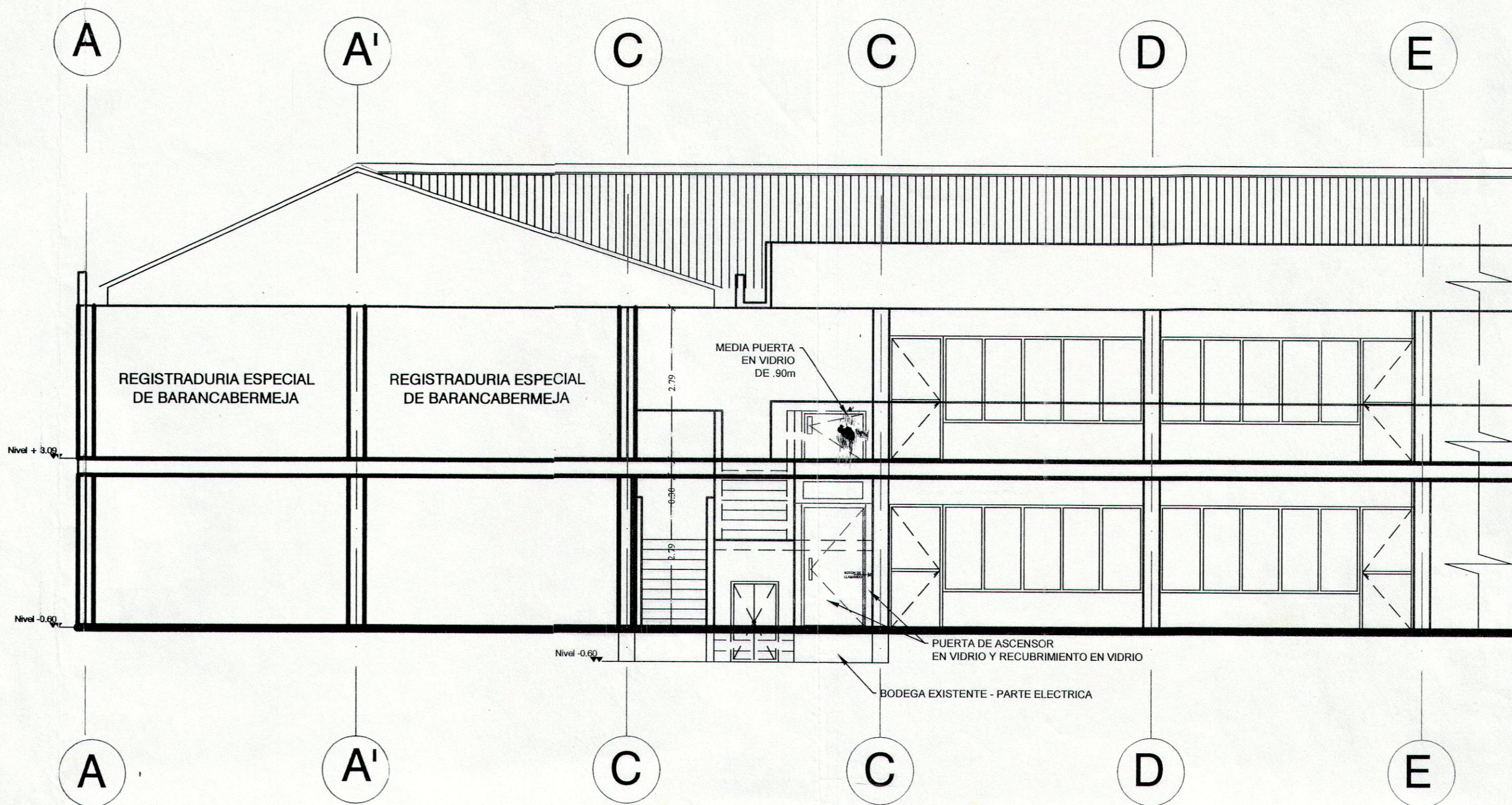
Corte F - F'
