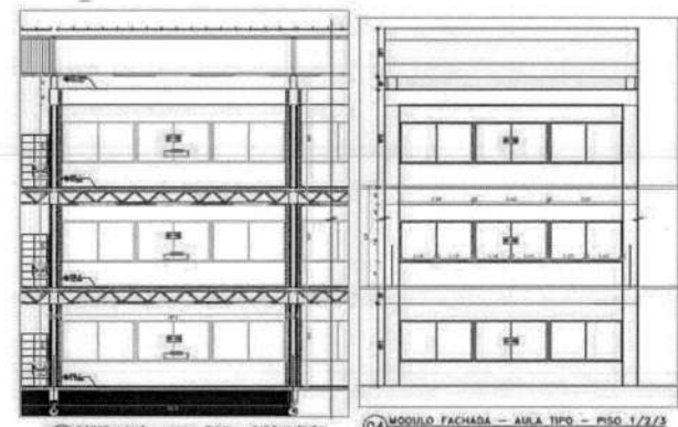
H CORTE LONGO - AULA TIPO - PISO 1/2/3
