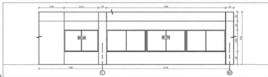
02 MODULO ELEVACION EXTERIOR - LABORATORIO TIPO - PISO 2
