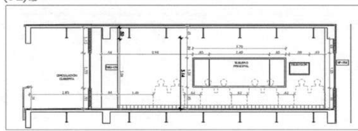
02 ELEVACION INTERIOR - AULA TIPO - PISO 2
