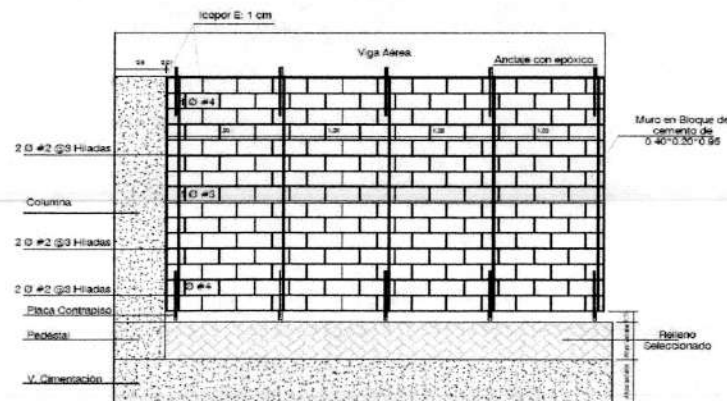
DETALLE DE REFUERZO DE MUROS
