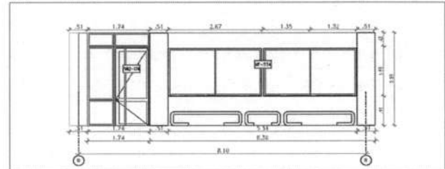
(02) ELEVACION INTERIOR - AULA TIPO - PISO 2
