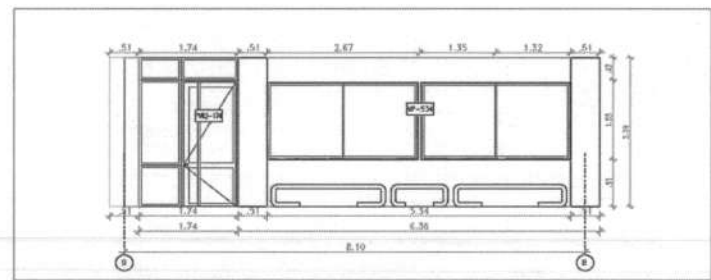
02 ELEVACION INTERIOR - AULA TIPO - PISO 2
