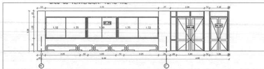
01 MODULO ELEVACION INTERIOR - LABORATORIO TIPO - PISO 2
