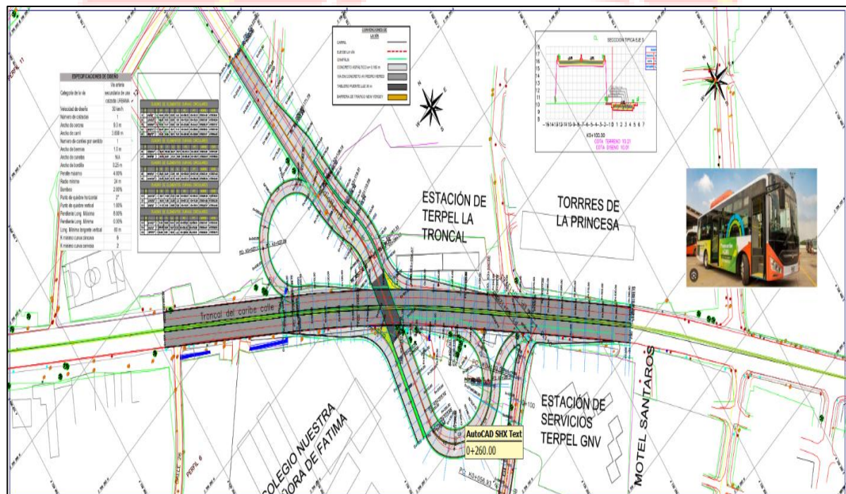
Imagen 3. Diseño Geométrico Aprobado.
