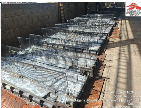
Ilustración 6. Desencofre y curado de paneles de concreto texturizado..
