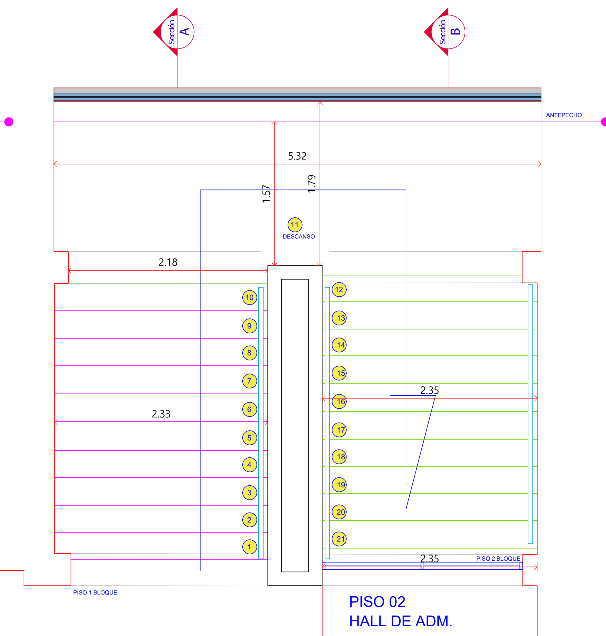
ESCALA 1:25
