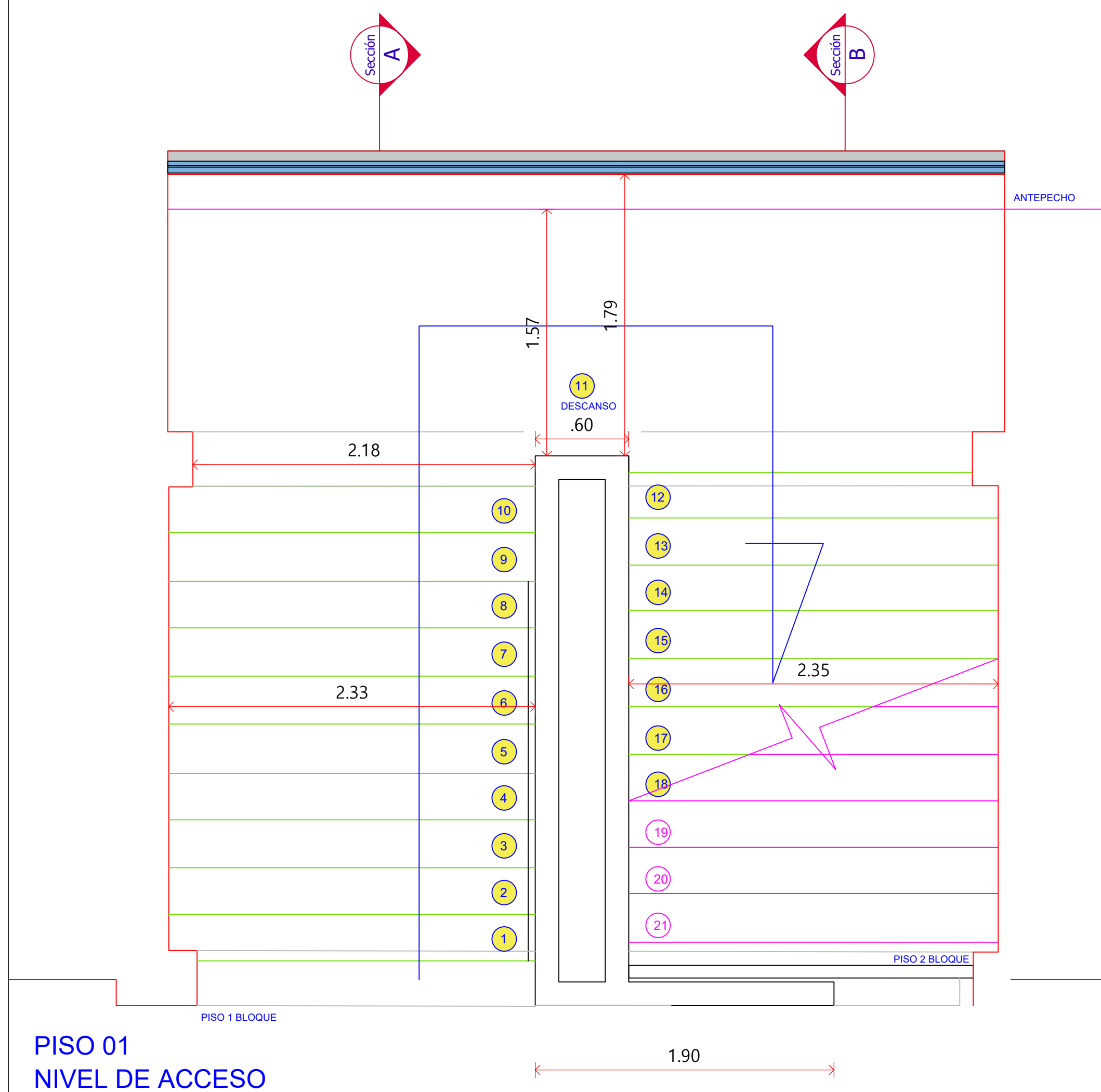
ESCALA 1:1000
