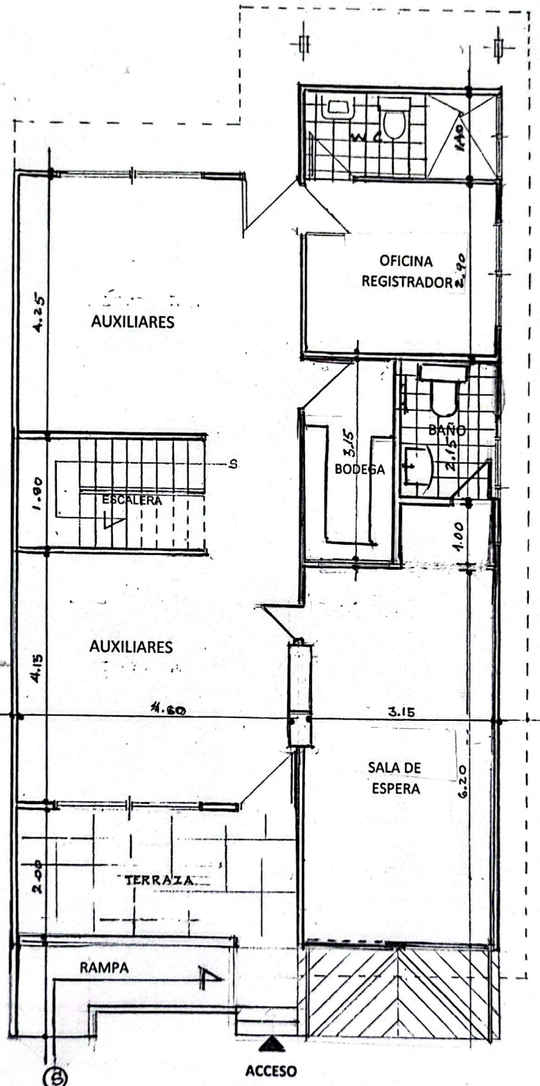
PLANTA PRIMER PISO ESCALA: 1-75
