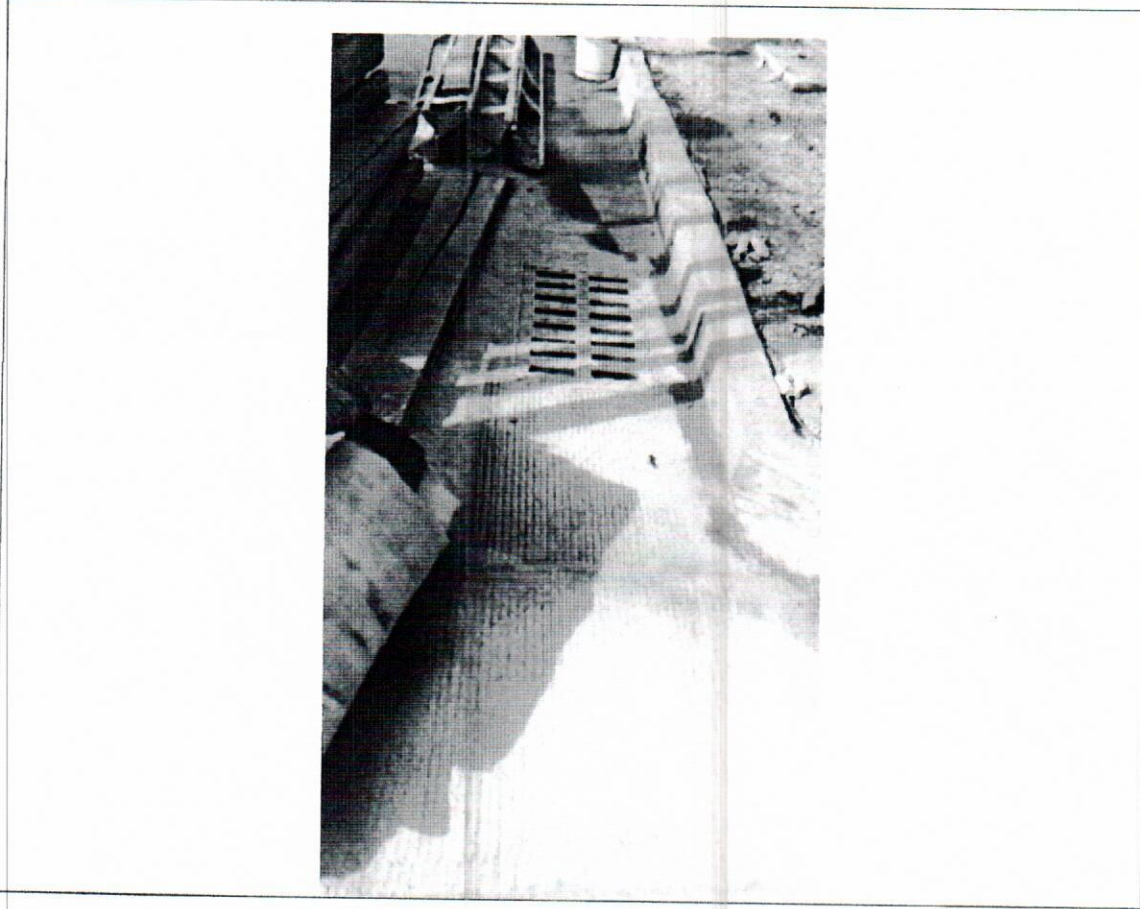
Sumidero lateral aguas lluvias en concreto reforzado de 21mpa con sello hidráulico, incluye rejilla en polipropileno
