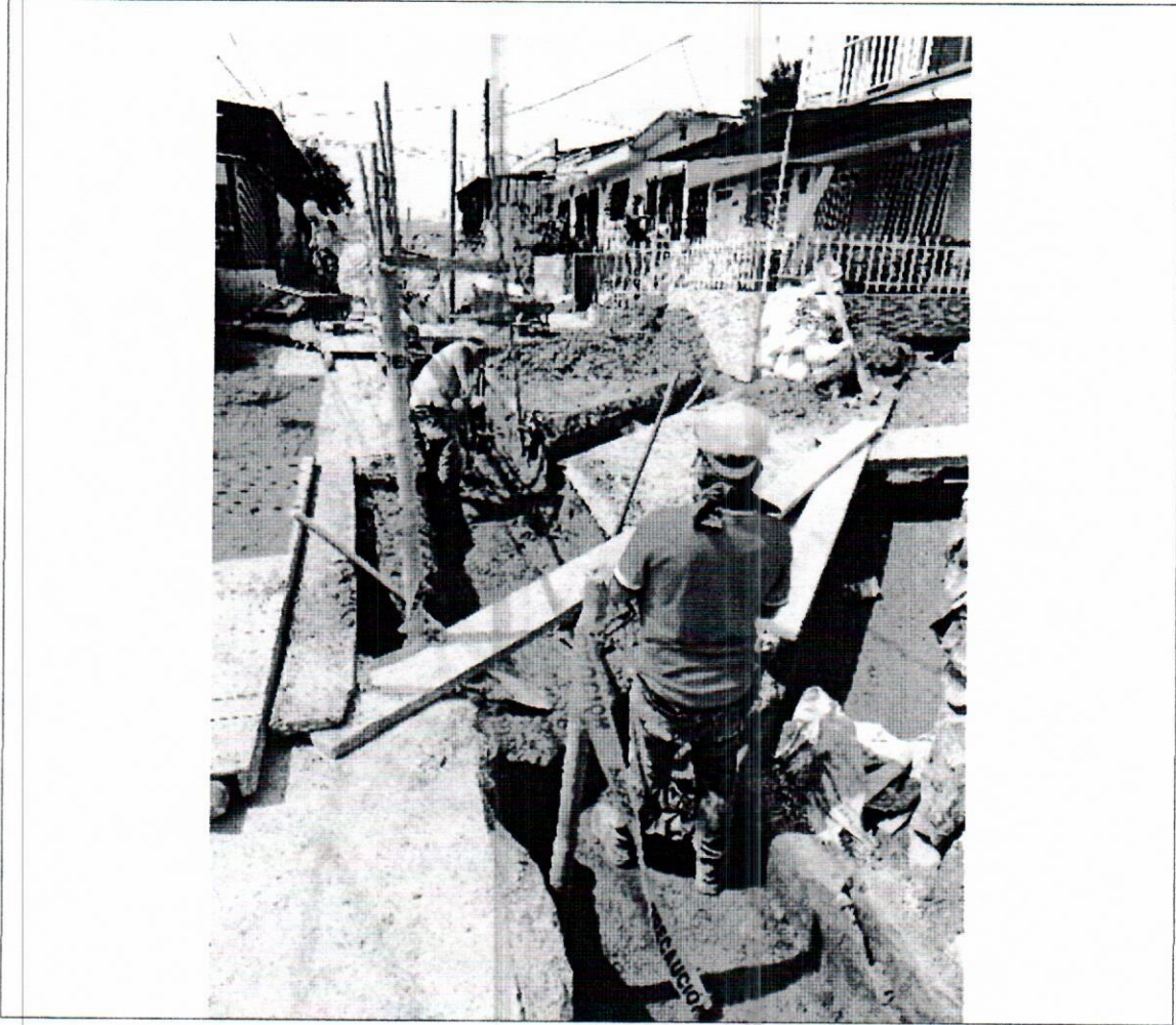
Llenos compactados
