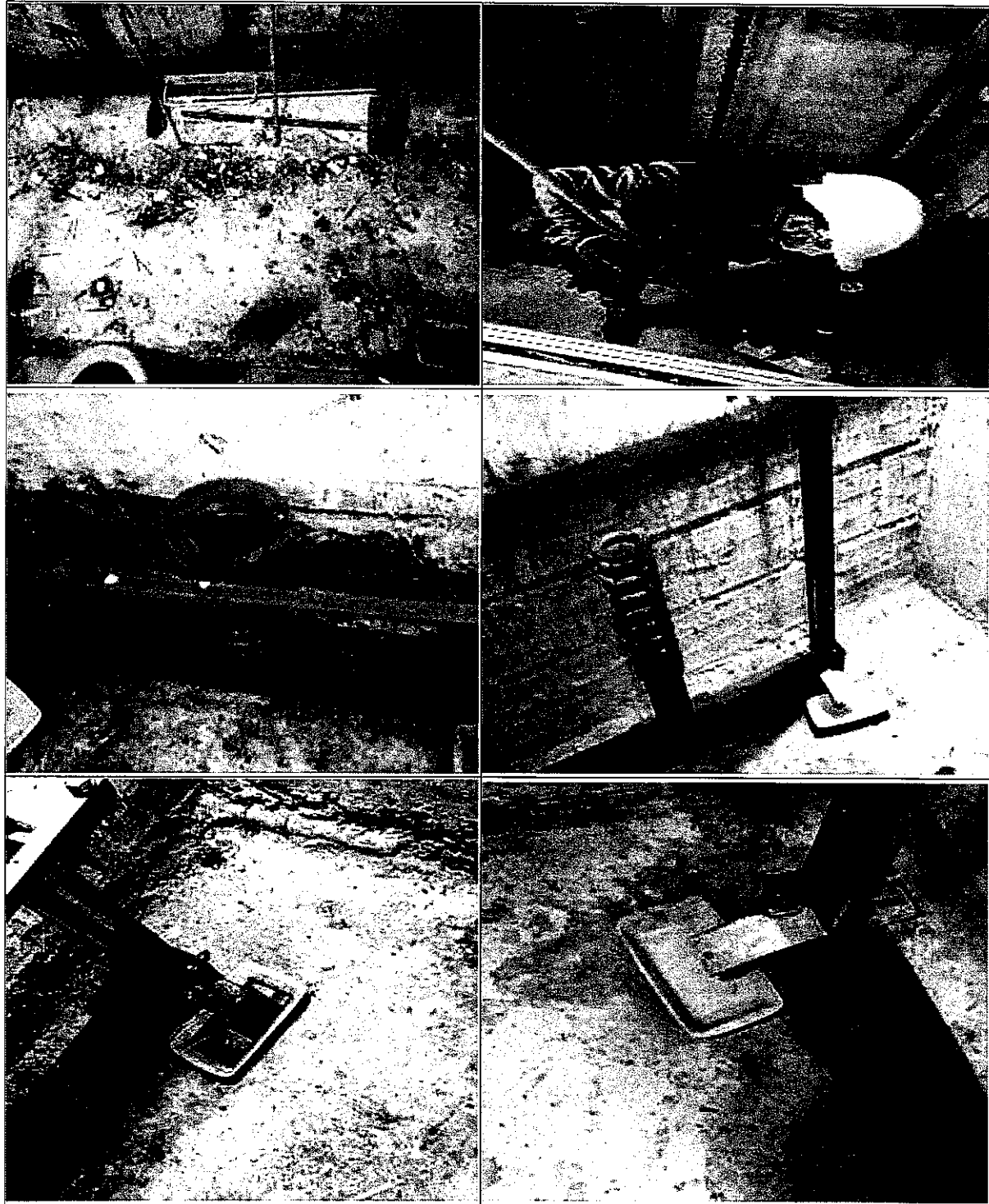
Ilustración 14: Verificación de operatividad al tablero de llamado en cabina (botoneras de cabina), revisión del estado de los sistemas de comunicación de emergencia, mantenimiento preventivo y limpieza a cada una de las condiciones en foso (buffers de cabina y contrapeso, aceiteras de cabina y contrapeso, verificación de la iluminación de foso, limpieza y lubricación de los rieles)
