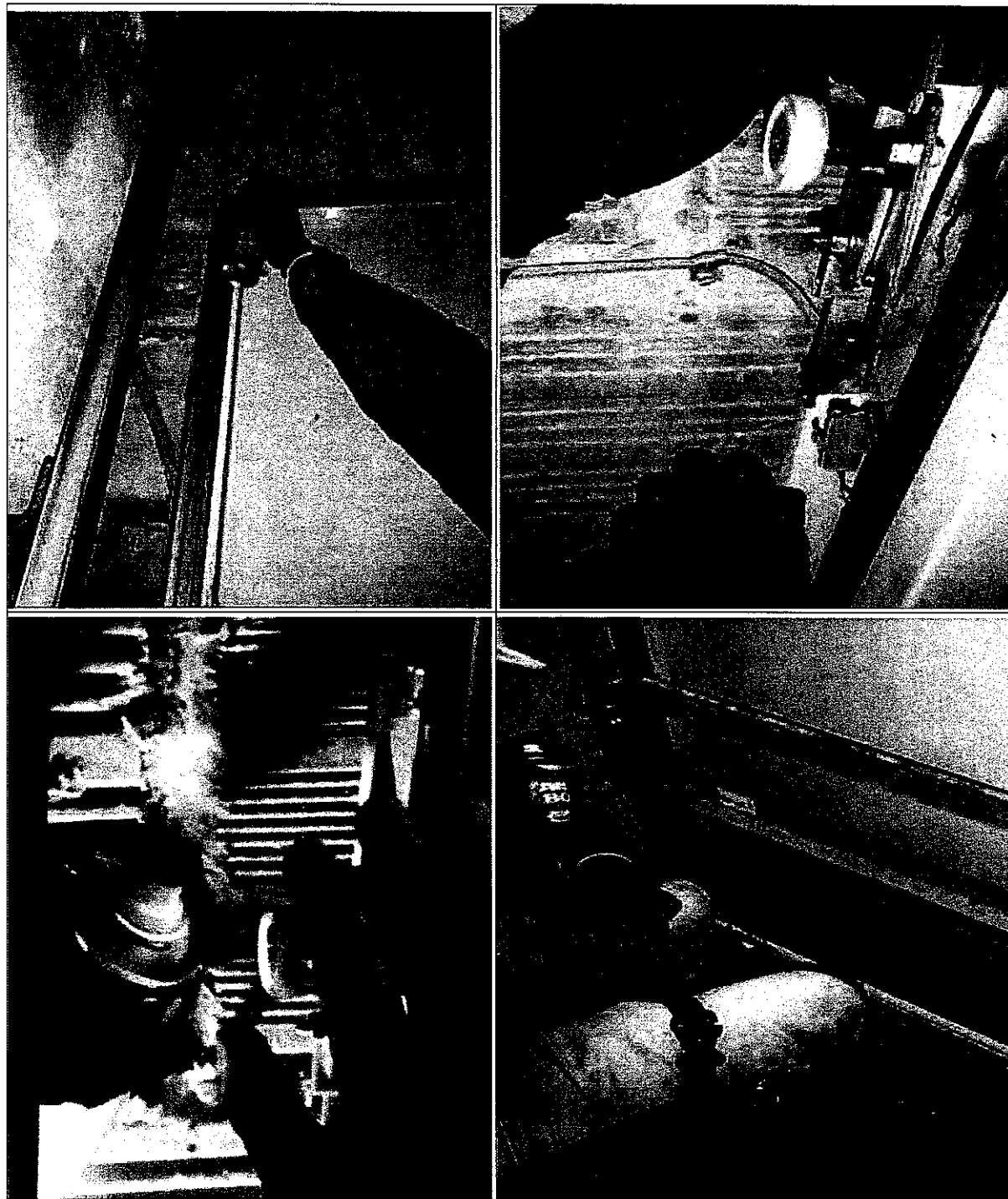
Ilustración 7: Mantenimiento preventivo, limpieza y lubricación a cada uno de los mecanismos de puertas de hall que conforman (correderas, excéntricas, guayas, topes, mantenimiento de rieles y micros de apertura) verificación a cada uno de los circuitos de aproximación de cierre de puertas.
