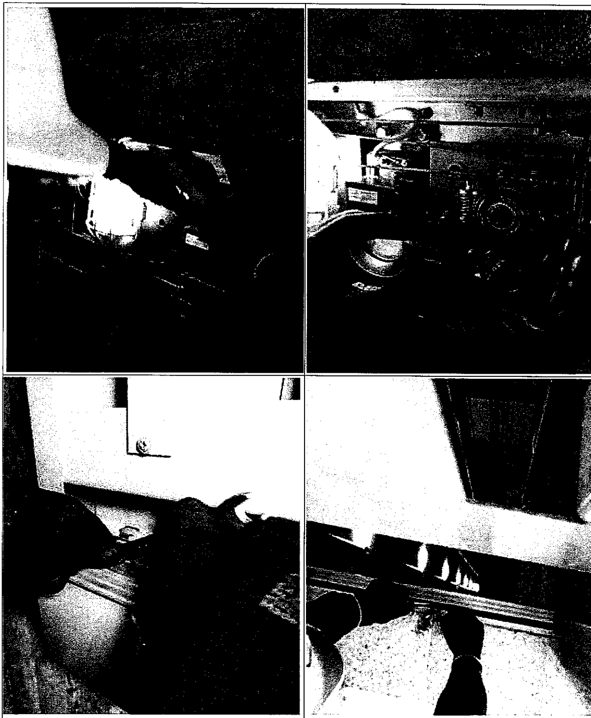
Ilustración 12: Mantenimiento preventivo limpieza y lubricación a cada uno de los mecanismos de apertura en puertas hall que conforman (correderas, zapatas, excéntricas, guías, contactos, resortes y guaya), verificación, cambio y ajuste de kit de zapatas para alinear y centrar las puertas hall, limpieza de quicios en cada piso.
