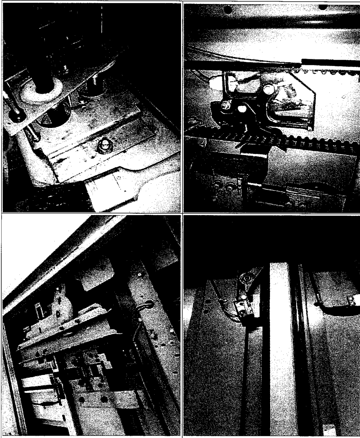
Ilustración 18: Mantenimiento preventivo, limpieza y lubricación a cada uno de los mecanismos de apertura y cierre en puertas de cabina que conforman (correderas, excéntricas, guías, contactos, resortes, poleas y guaya).
