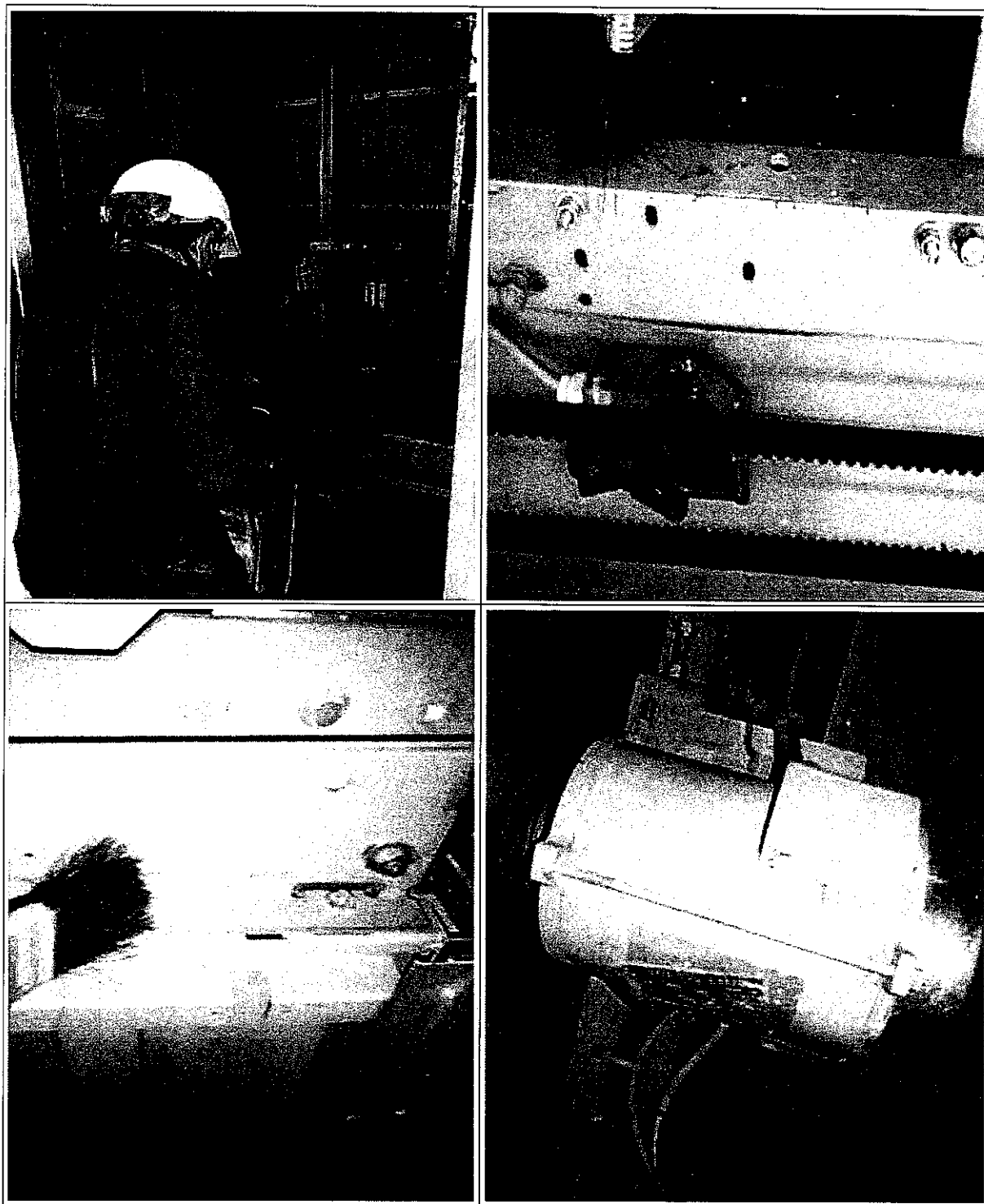
Ilustración 13: Mantenimiento preventivo, limpieza y lubricación a cada uno de los mecanismos de apertura y cierre en puertas de cabina, limpieza y lubricación a los ventiladores de cabina, verificación y ajuste a las hojas, a la correa de tracción y alineación de las bandas de rayos múltiples RX (emisor y receptor).
