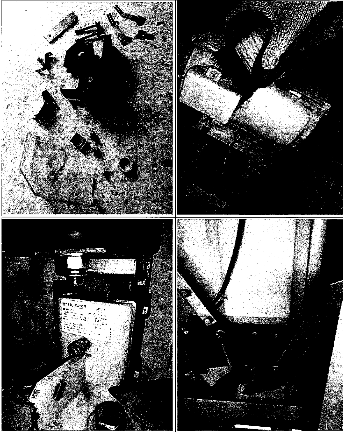
Ilustración 23: Revisión del sistema eléctrico de alimentación sobre cabina, ajuste a la correa del motor de apertura de puertas de cabina, limpieza de quicios y lubricación de los mecanismos (rolletes, excéntricas, rodamientos)
