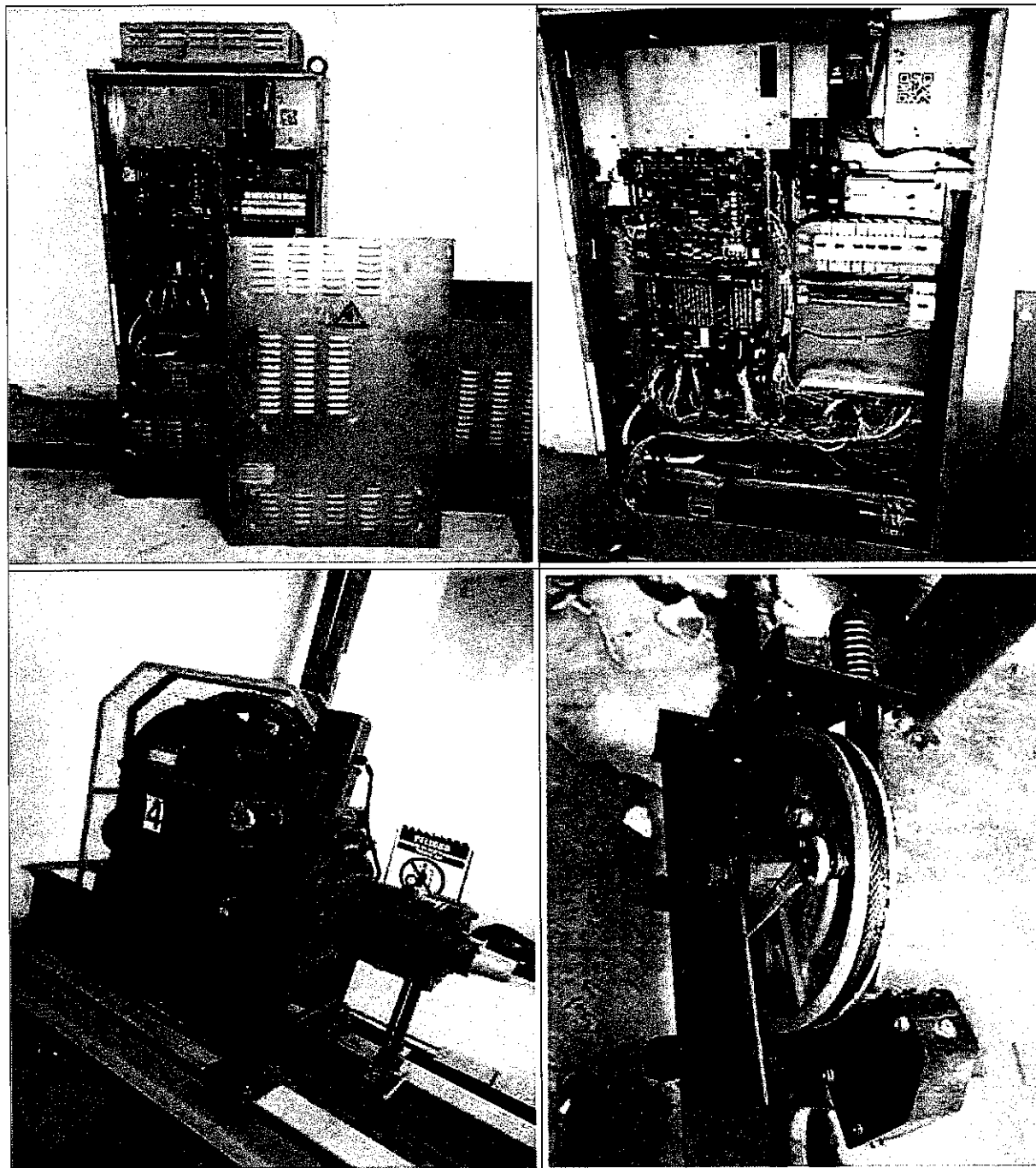
Ilustración 10: Revisión a cada uno de los componentes generales en cuarto de máquinas (motor, polea deflectora y revisión de electro freno, limitador de velocidad (gobernador)), verificación eléctrica del sistema de alimentación, verificación del nivel de aceite, verificación de cables de tracción y a cada elemento del cuadro de control principal.
