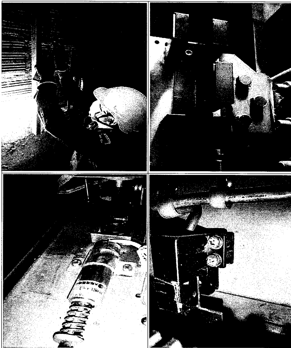
Ilustración 16: Mantenimiento preventivo limpieza y lubricación a cada uno de los componentes que conforman (límites superiores e inferiores, prefinales, inductor de aproximación) verificación a las fuentes de alimentación de las botoneras de hall, limpieza y lubricación a los ventiladores en cabina.
