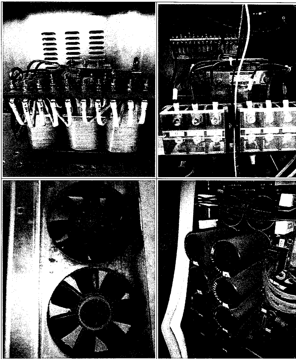
Ilustración 26: Mantenimiento preventivo y limpieza a cada uno de los circuitos eléctricos de cuadro de control principal (transformadores, banco de condensadores, ventiladores disipadores, tarjeta de potencia), verificación de voltaje a cada uno de los circuitos de alimentación, revisión de las fases de los transformadores de sobre tensión.
