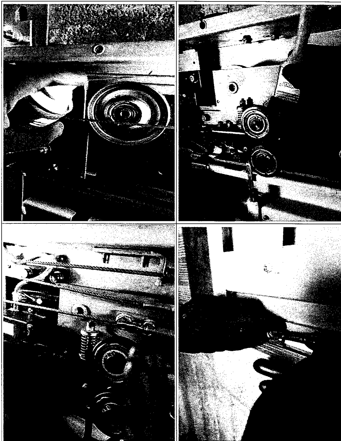
Ilustración 27: Mantenimiento preventivo limpieza y lubricación a cada uno de los mecanismos de apertura en puertas hall y de cabina que conforman (correderas, excéntricas, guías, contactos, resortes, poleas y guaya), cambio kit de zapatas ajuste y calibración.
