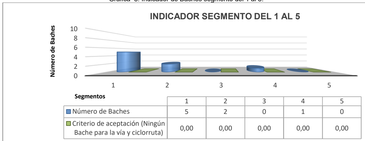
Gráfica 5. Indicador de Baches segmento del 1 al 5.
