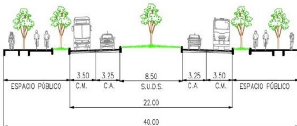
Ilustración 1 Secciones Típicas de las Unidades Funcionales - (c) sección típica de la UF6.
