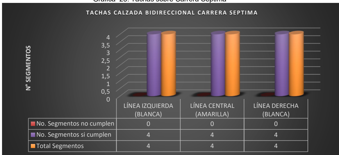
Gráfica 23. Tachas sobre Carrera Séptima
