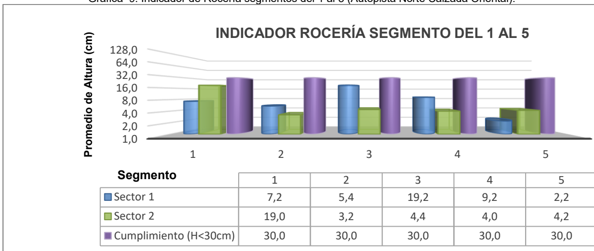
Gráfica 9. Indicador de Rocería segmentos del 1 al 5 (Autopista Norte Calzada Oriental).
