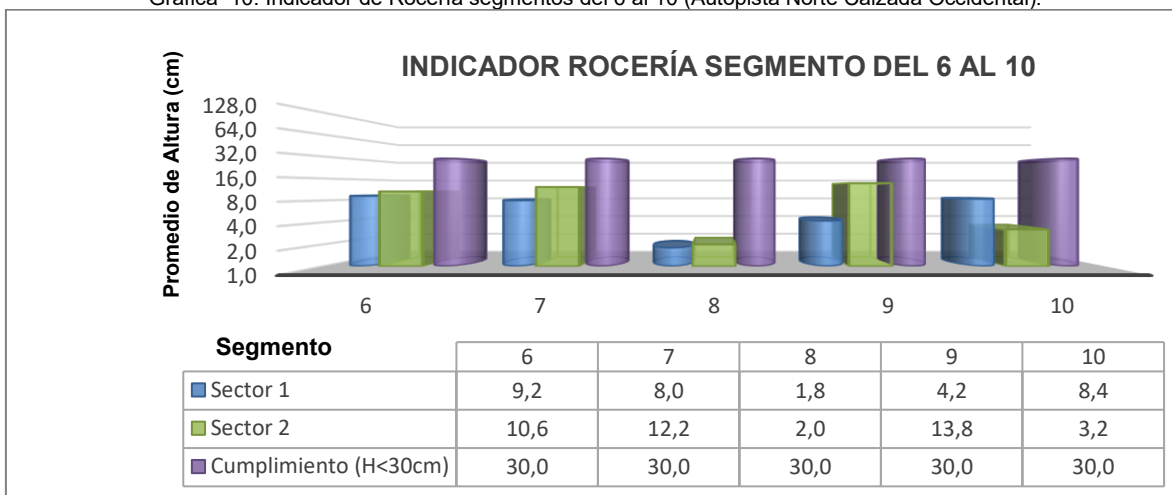
Gráfica 10. Indicador de Rocería segmentos del 6 al 10 (Autopista Norte Calzada Occidental).
