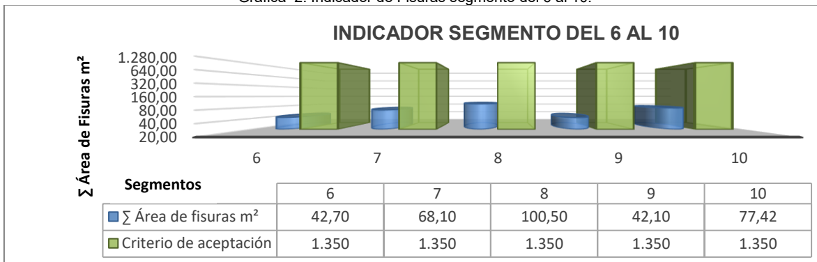
Gráfica 2. Indicador de Fisuras segmento del 6 al 10.
