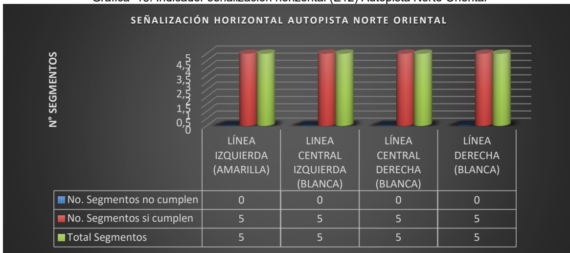
Gráfica 18. Indicador señalización horizontal (E12) Autopista Norte Oriental
