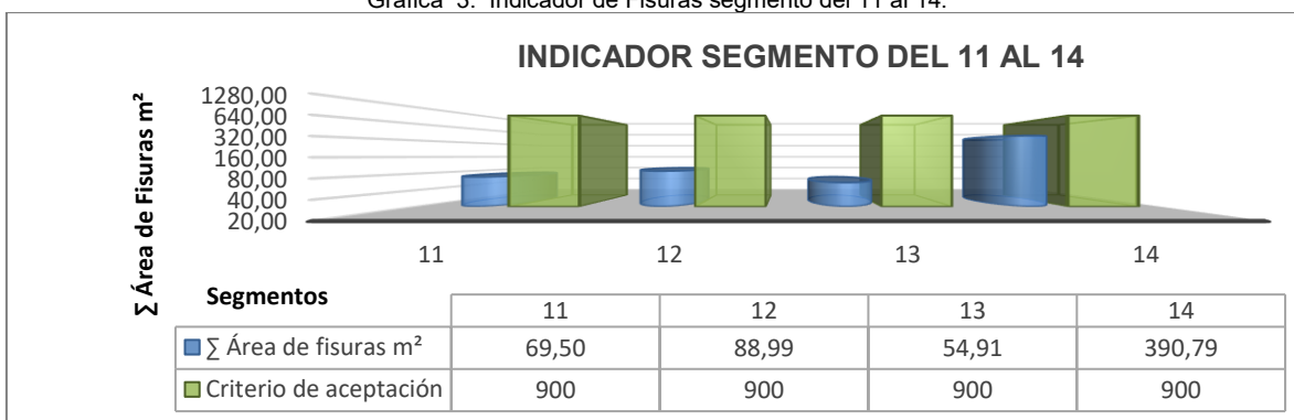
Gráfica 3. Indicador de Fisuras segmento del 11 al 14.
