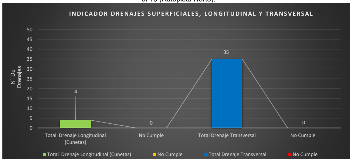
Gráfica 14. Resumen indicador, Drenajes superficiales, longitudinales y transversales (E10) Segmentos del 1 al 10 (Autopista Norte).
