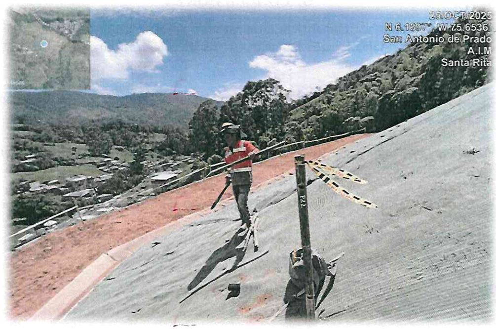
Piezómetro 2 (PZ-2)
