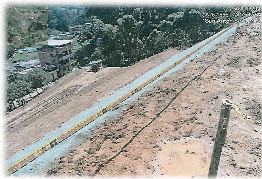
Inclinómetro 2 (INCL-2)
