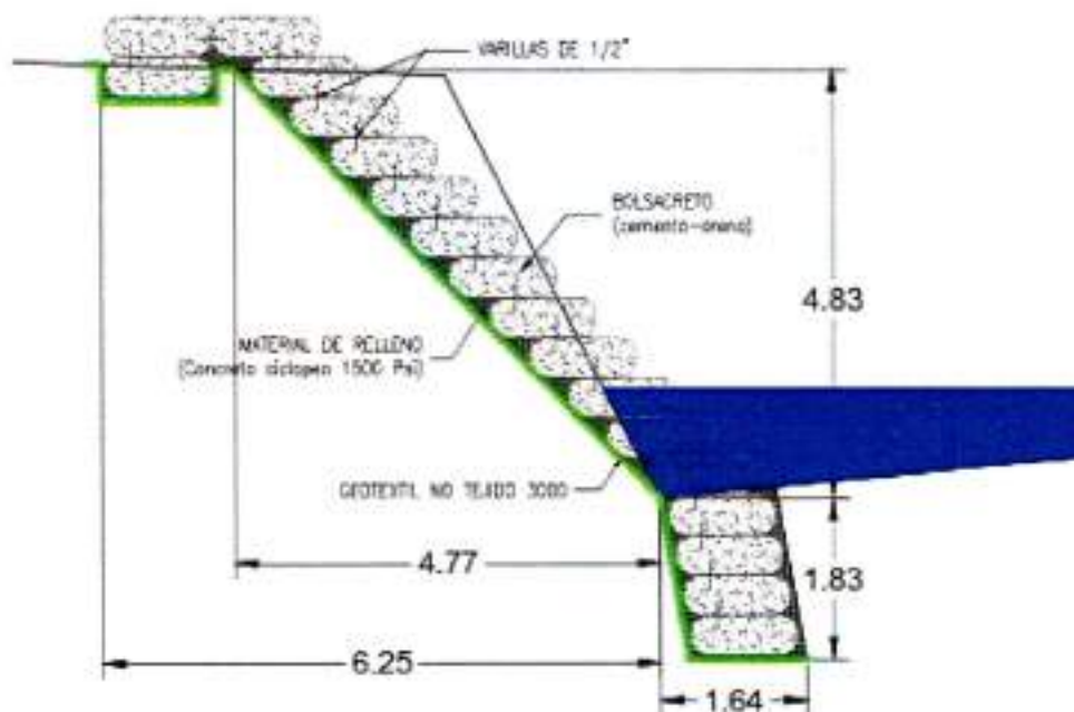
Ilustración 5. CORTE OBRAS DE PROTECCION LATERAL
