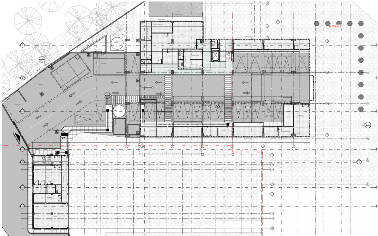
Planta Cubiertas
