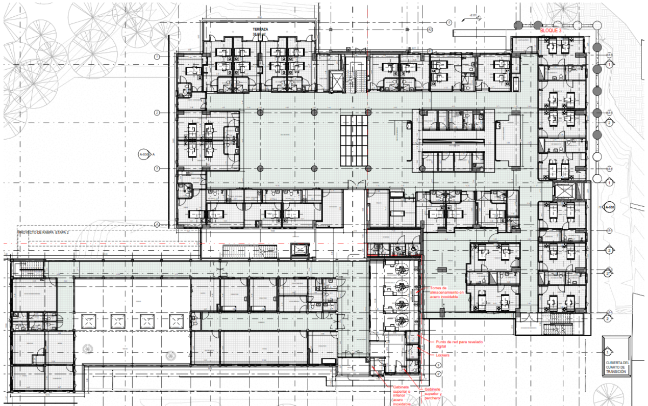
Planta nivel 3
