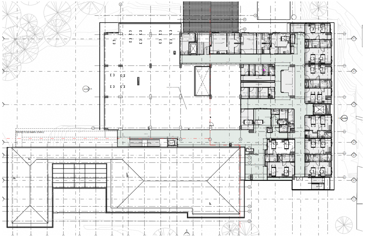
Planta nivel -1
