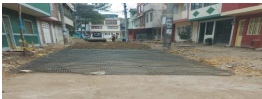
Instalación de geomalla y primera capa de material AR-BG38 estabilizado CIV 8009549 (NC28).
