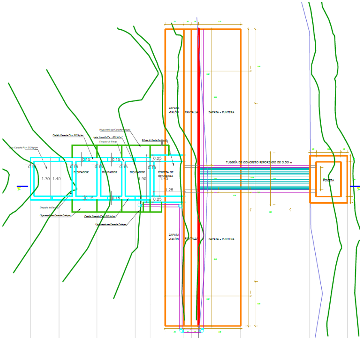
Planta muro alcantarilla y descole o dissipador de energía
