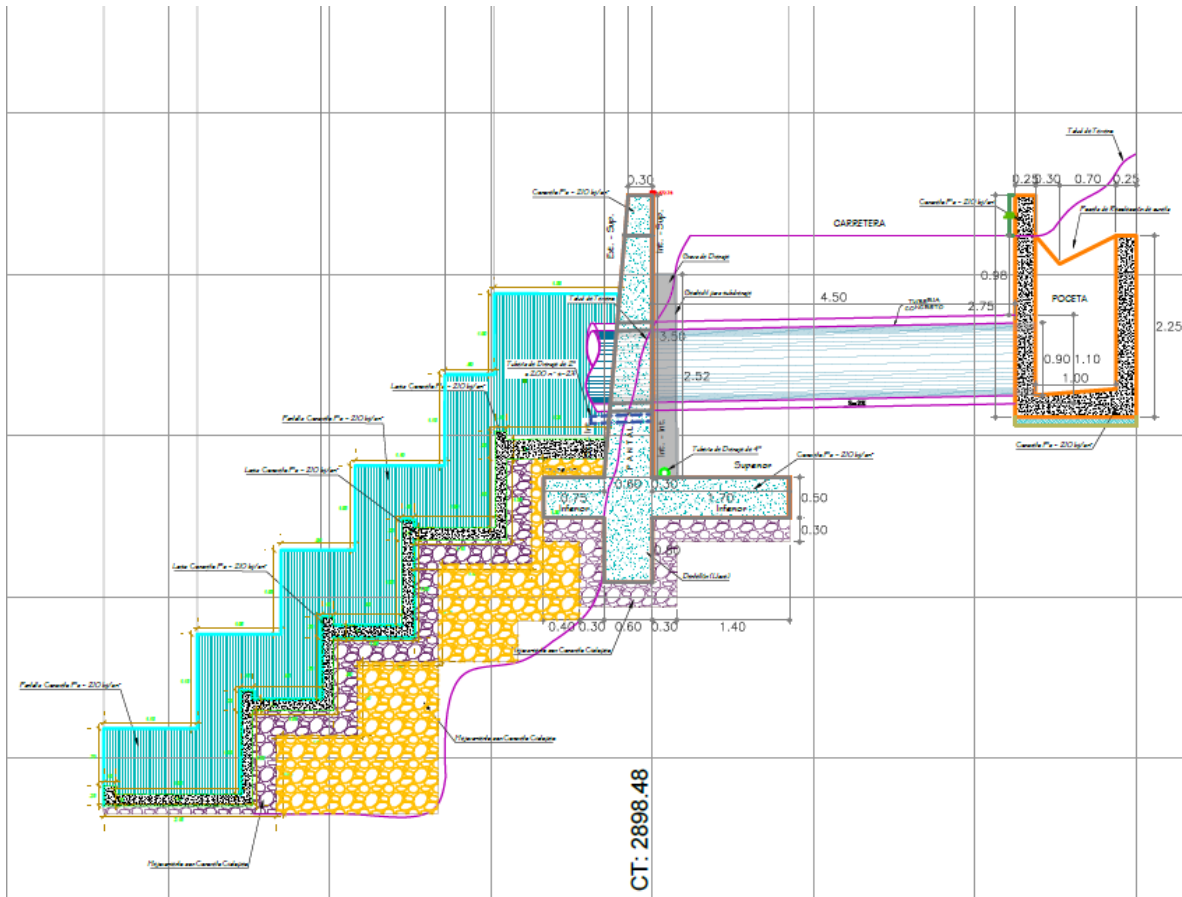
Perfila muro alcantarilla
