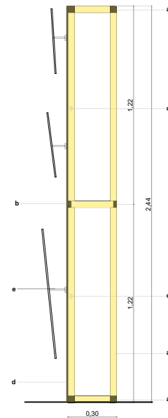
Sección Tipo Esc 1:10
