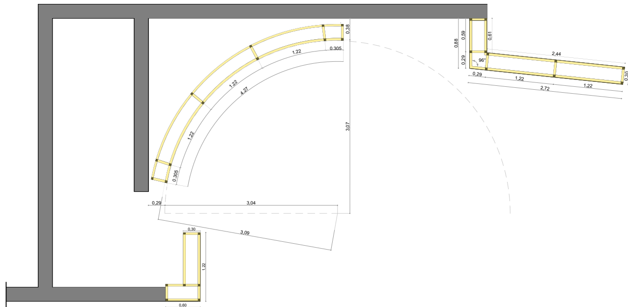
Plano Esc 1:20
