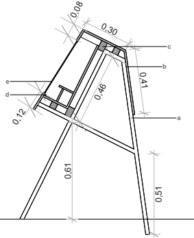
Sección Esc 1:10
