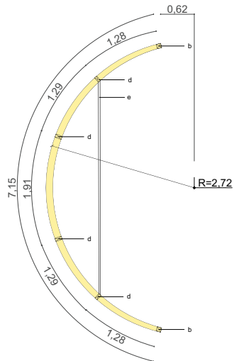
Planta Cabina Leo Radio Esc: 1:30
