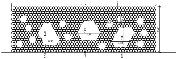
Alzado Muro Librería Esc 1:30
