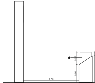
Alzado Muro Mapa Esc 1:50
