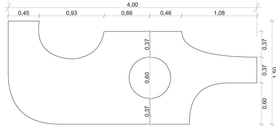
Planta Esc 1:20
