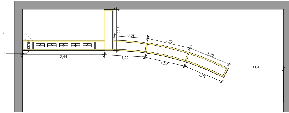
Planta Muro Interactivo Esc 1:20
