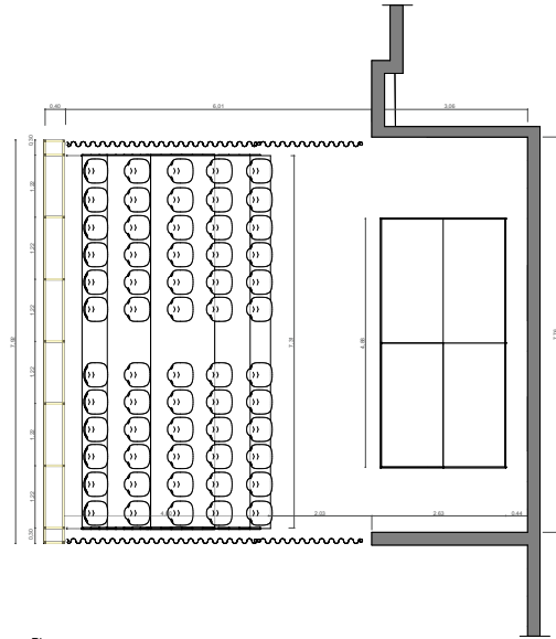
Plano Esc 1:50
