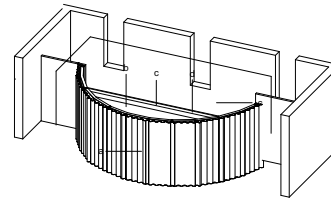
Axonometría
