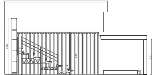
Sección Esc 1:50
