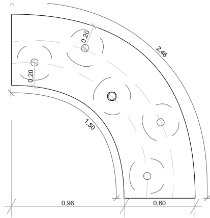
Planta Esc 1:50
