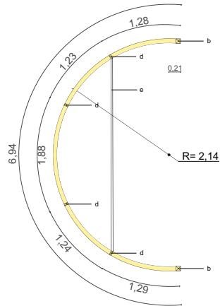
Planta Cabina Acoger la Escucha Esc: 1:30
