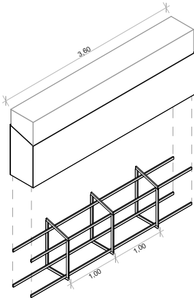
Axonometría
