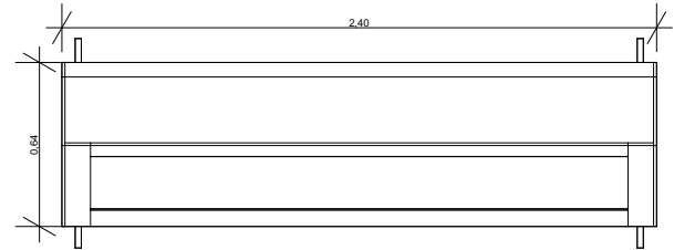
Planta Esc 1:10
