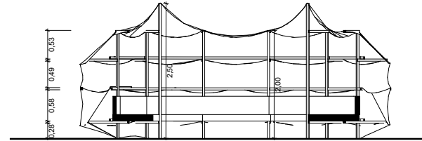
Alzado Módulo Lectura Esc 1:30
