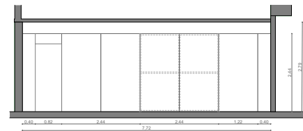
B. Muro en Triplex oficinas y bodega Escala 1:50
