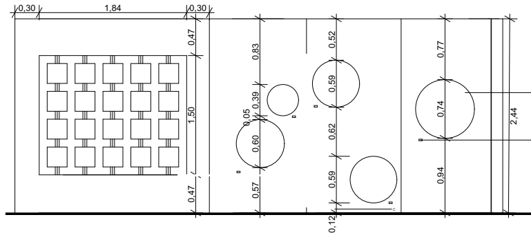
Alzado Muro Interactivo Esc 1:20
