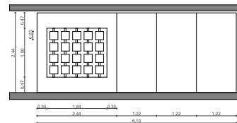
F. Muros Muro Interactivo Escala 1:50
