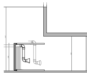
Sección Esc: 1:50
