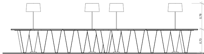
Alzado Esc 1:20
