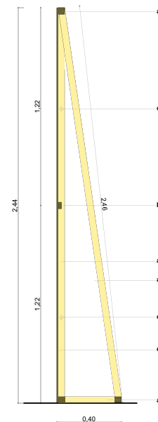
Sección Esc 1:50
