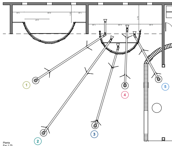
Planta Esc: 1:75
