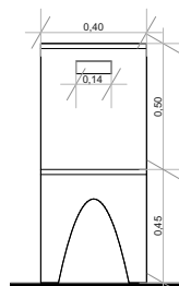
Alzado frontal Esc 1:10
