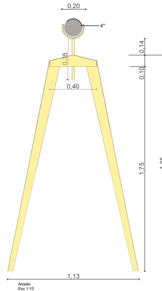
Alzado Esc: 1:10
