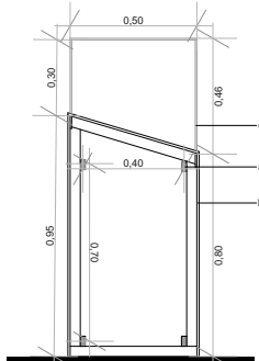
Sección Esc 1:10
