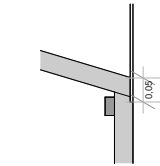
Detalle Empate Vidrio Esc 1:5
