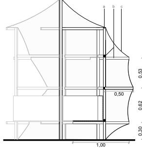
Detalle Módulo Lectura Esc 1:20
