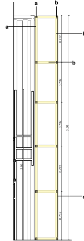
Sección Detalle muro Mapa Esc 1:20
