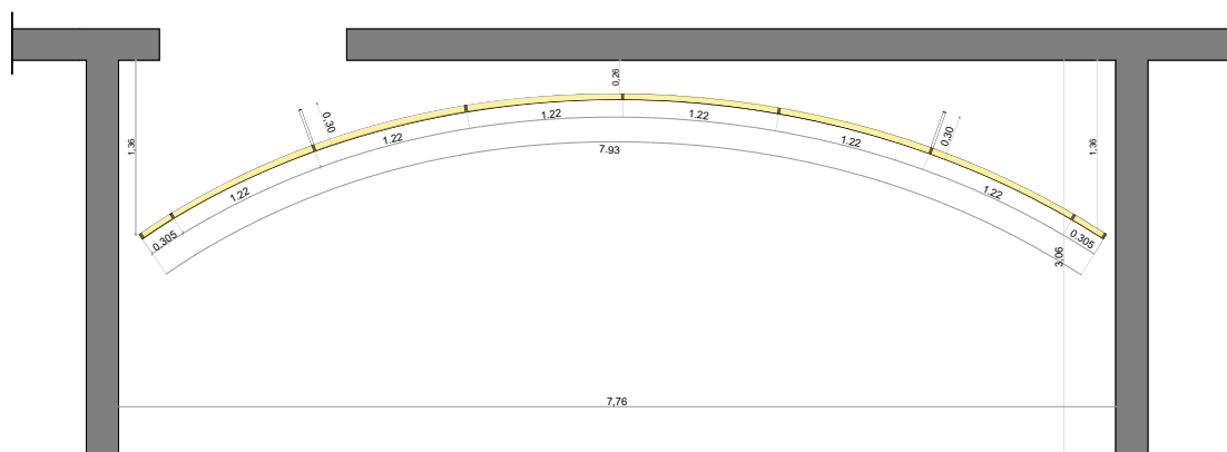
Plano Esc 1:50
